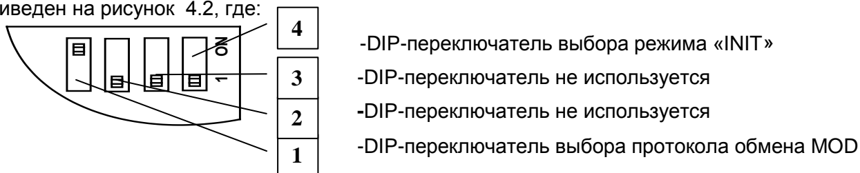
Рисунок 4.2 - BUS RTU.
