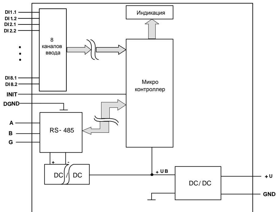
Рисунок 4.2 – Функциональная схема модуля DI-8H
