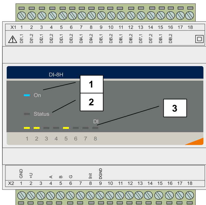
Рисунок 4.1 – Вид модуля со стороны передней панели
