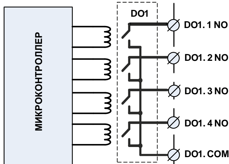
Рисунок 5.2 – Первая группа релейных каналов вывода
