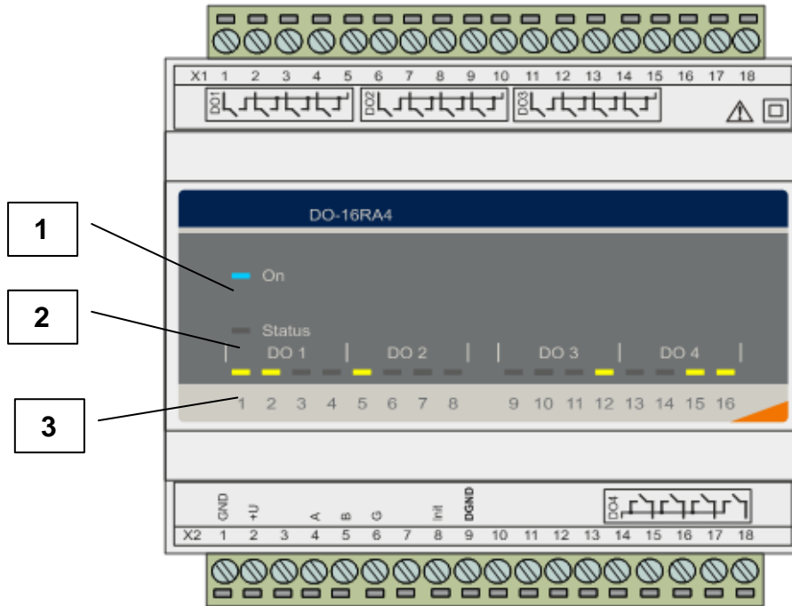
Рисунок 4.1 – Вид модуля DO-16RA4 со стороны передней панели
