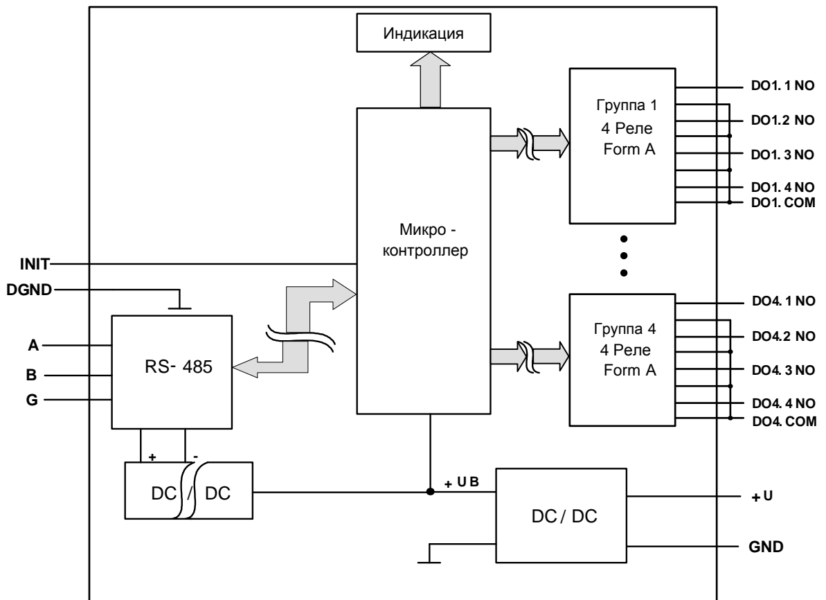
Рисунок 4.2 – Функциональная схема модуля DO-16RA4
