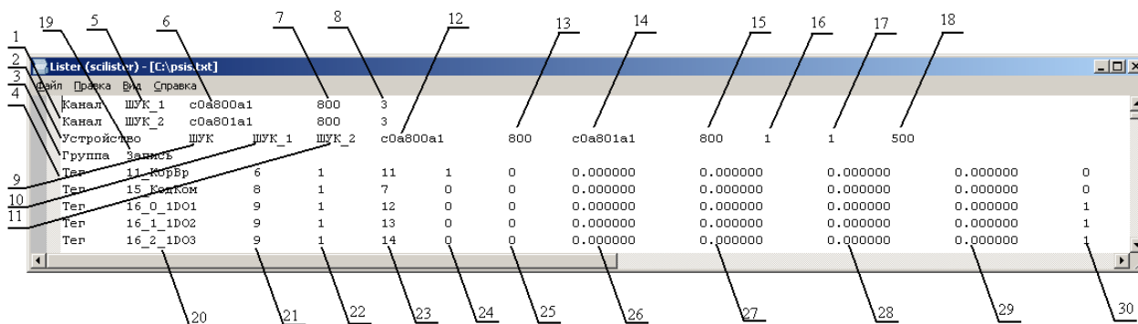
Рисунок 6.7 – Файл psis.txt
