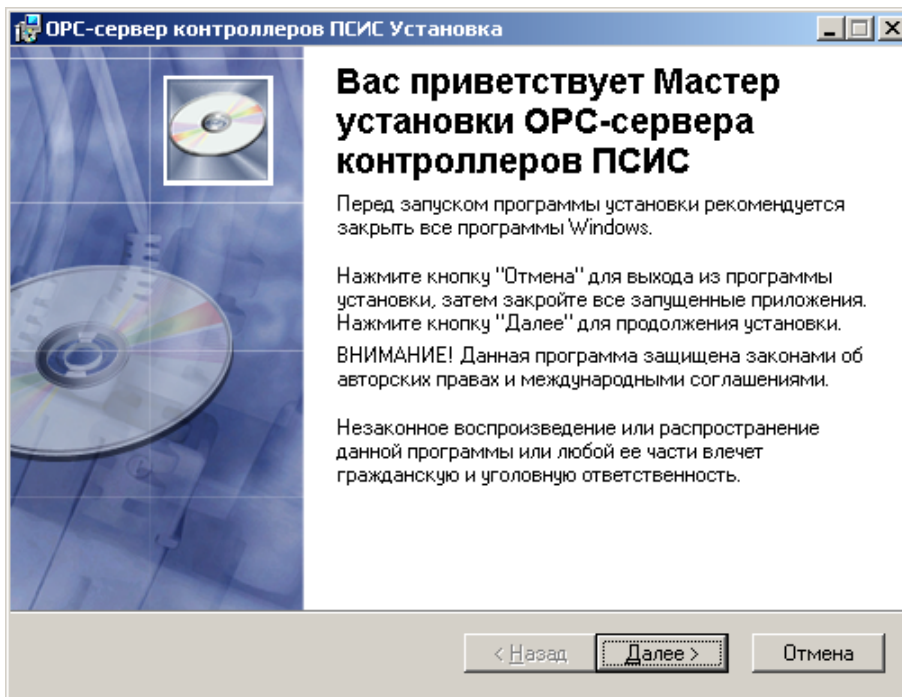
Рисунок 3.1 - Окно инсталлятора
