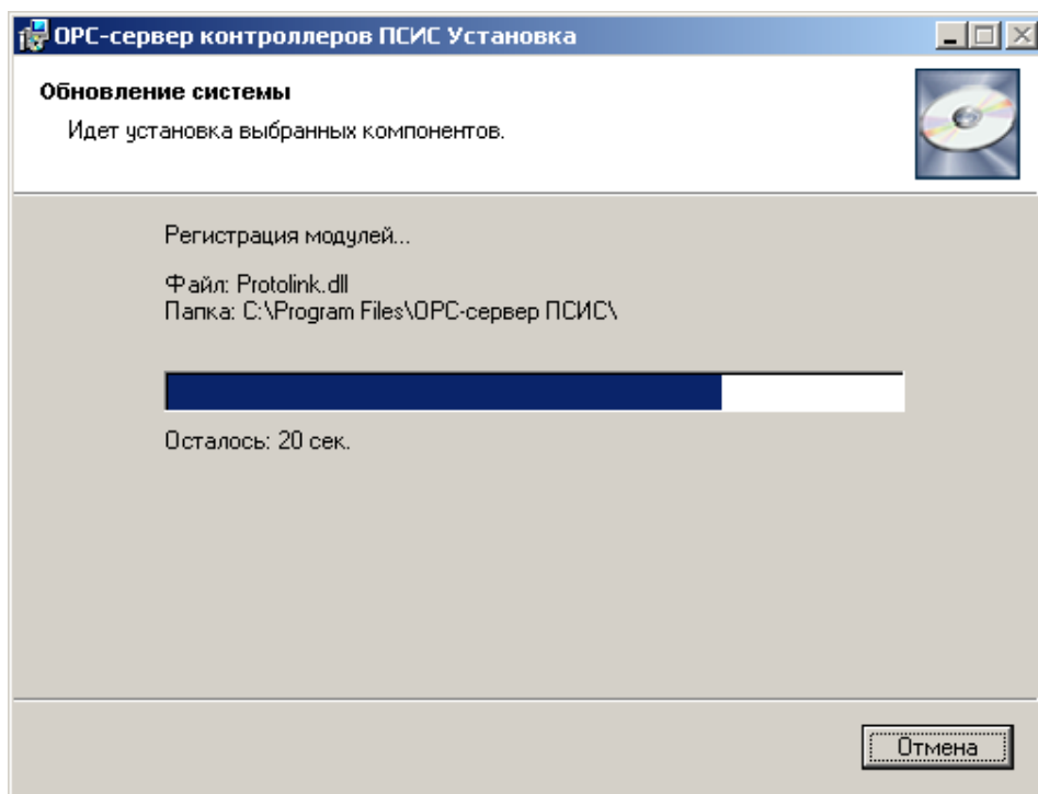
Рисунок 3.5 - Копирование файлов
