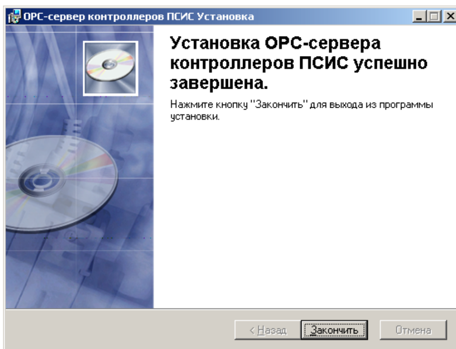
Рисунок 3.6 - Установка завершена
