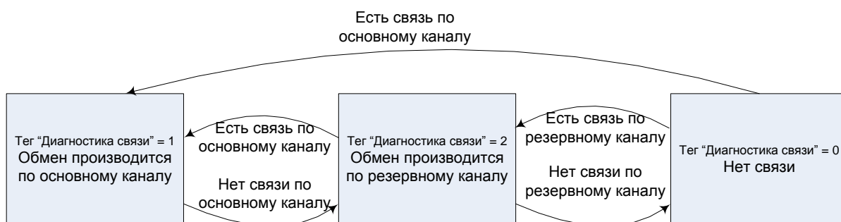
Рисунок 6.8 – Схема работы резервирования каналов
