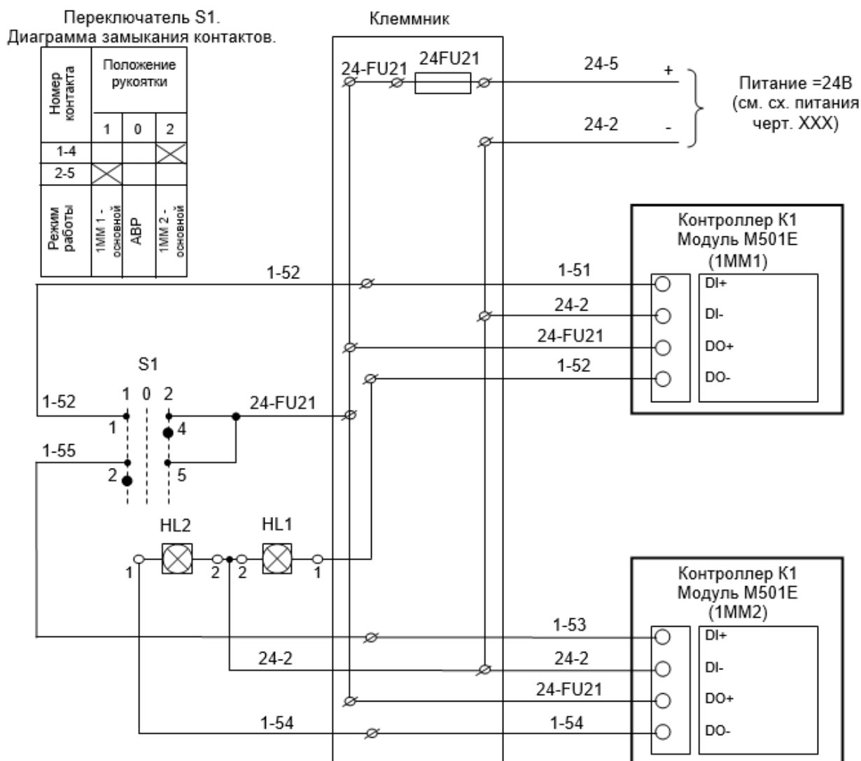
Рисунок 4.1.4.3.5 – Пример схемы резервирования №2 при резервировании процессорных модулей контроллера TREI-5B-05 Smart TP
