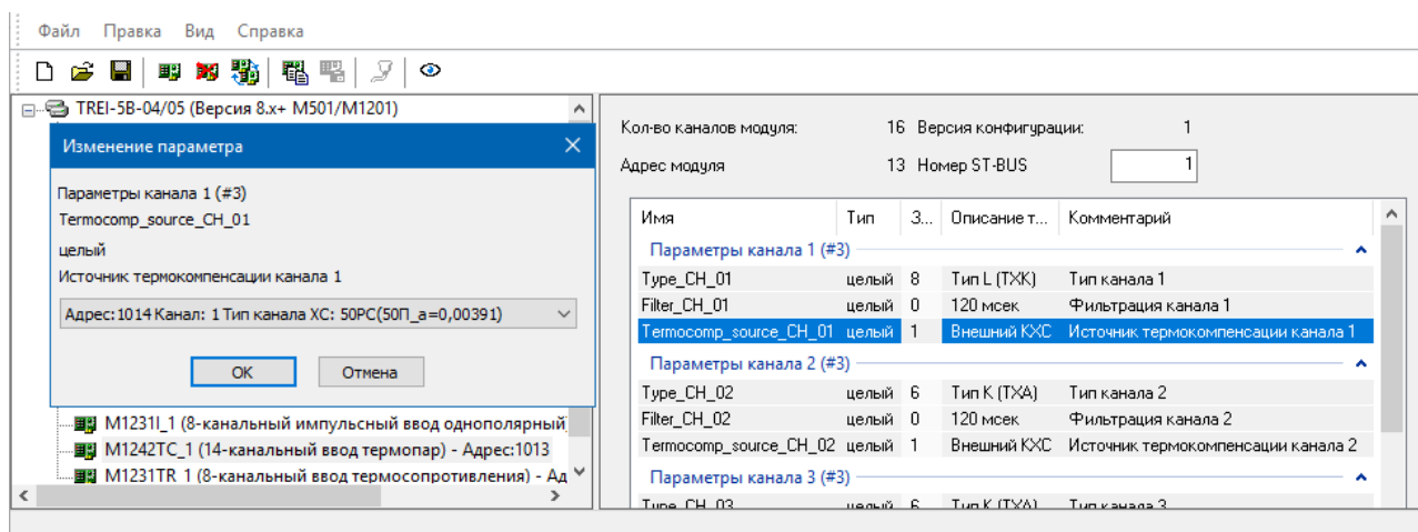
Рисунок В.12.1 – Назначение источника термокомпенсации
