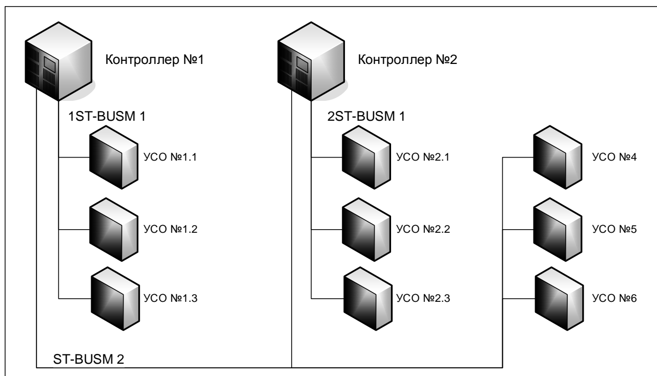
нок 4.1.4.4.1 – Структура со «смешанным» резервированием контроллеров TREI-5B-04
