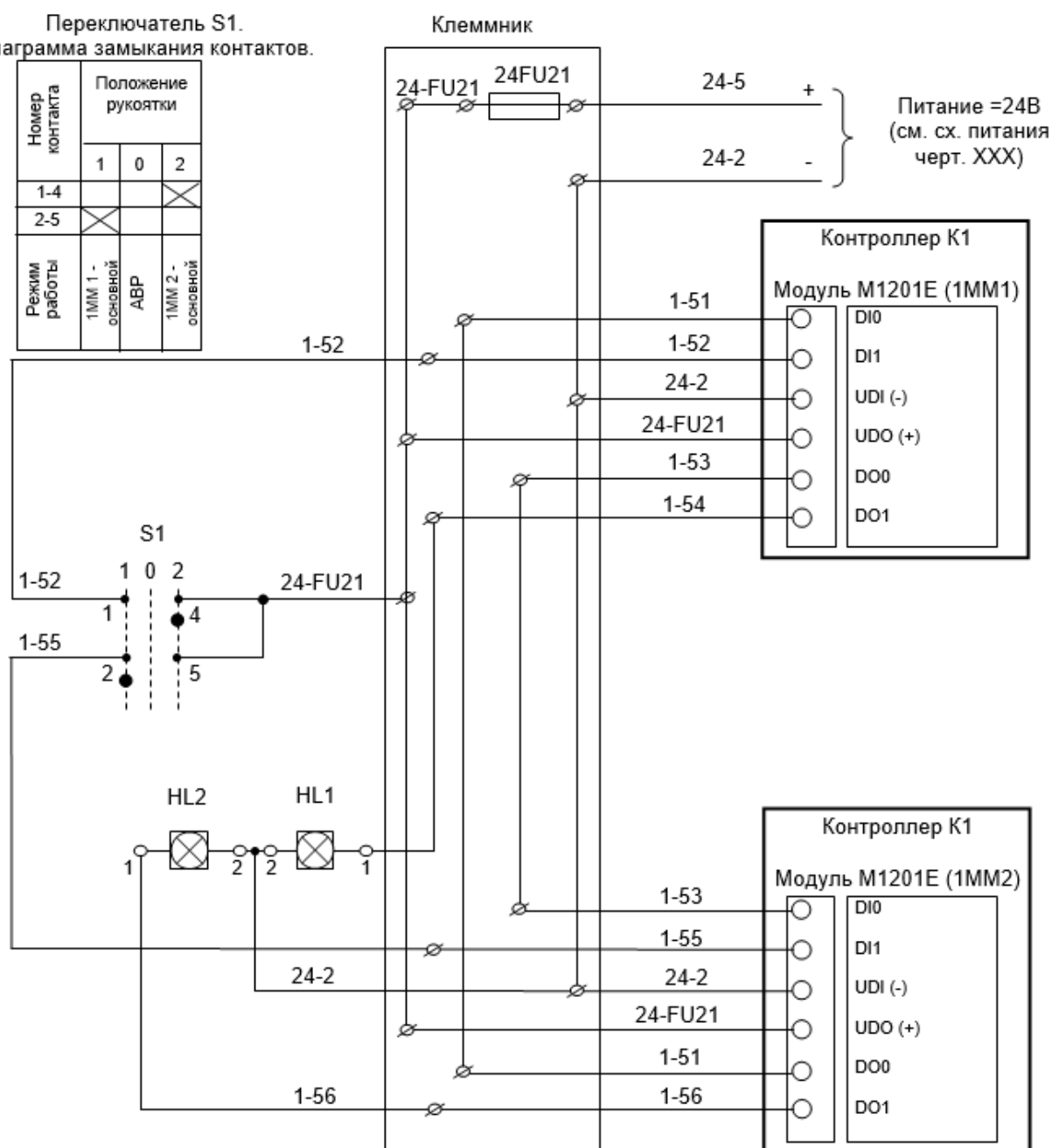
Рисунок 4.1.4.3.1 – Пример схемы резервирования №0 при резервировании процессорных модулей контроллера TREI-5B-04 STANDARD
