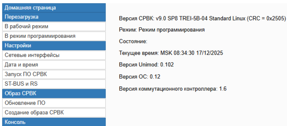
Рисунок Д.2 – Главная страница
