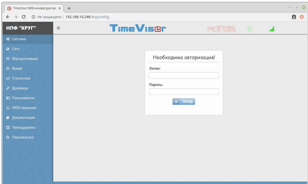
Рисунок 5.2 – Страница авторизации
