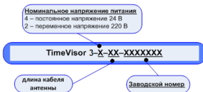
Рисунок 3.2 – Условное обозначение СЕВ «TimeVisor3»
