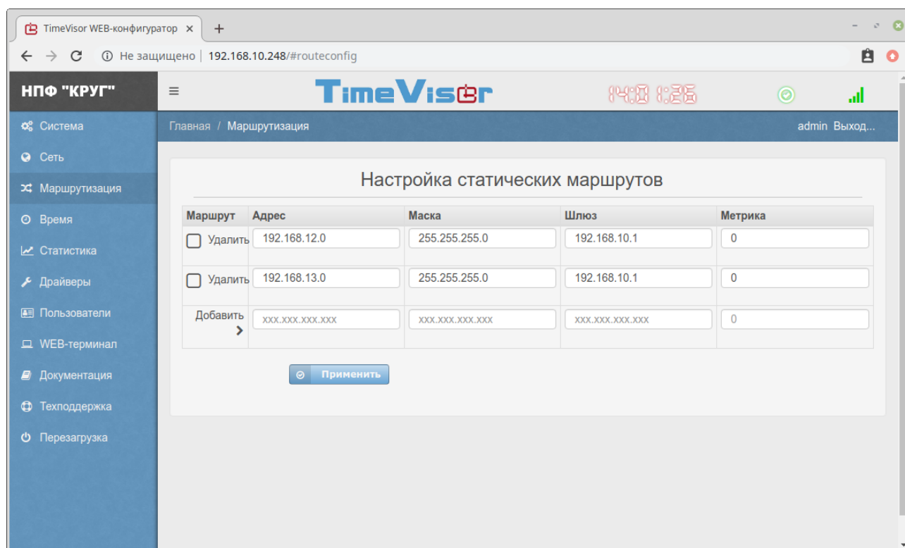
Рисунок 5.5 – Страница «Настройка статических маршрутов»
