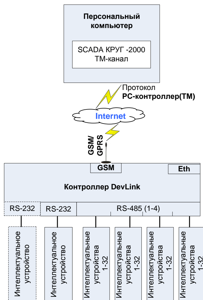
Рисунок 5.7 – Схема передачи данных в SCADA КРУГ-2000 по сети Internet
