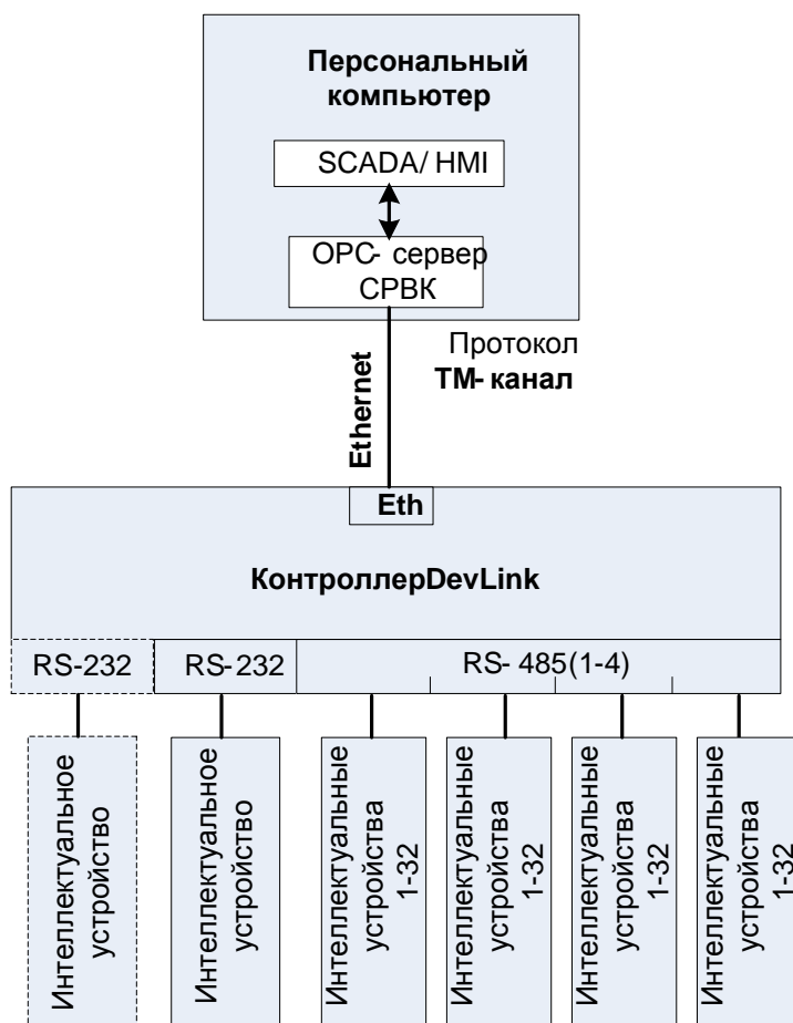
Рисунок 5.2 – Схема передачи данных по сети Ethernet по протоколу TM-канал
