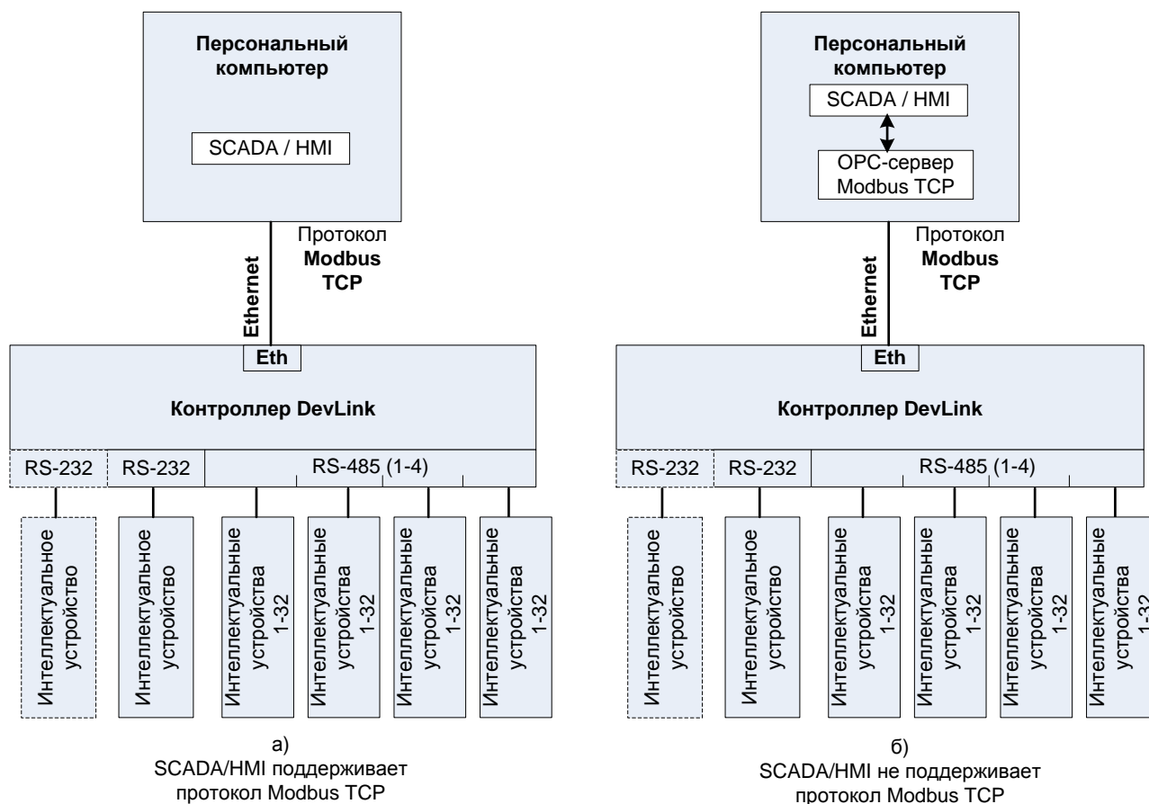
Рисунок 5.1 – Схема передачи данных по сети Ethernet по протоколу Modbus TCP
