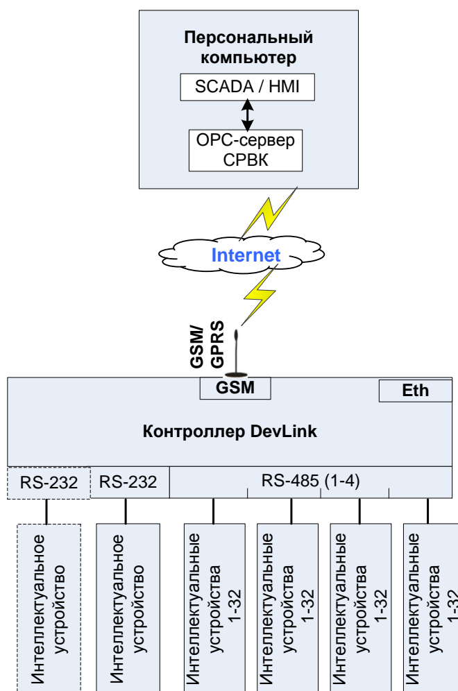
Рисунок 5.6 – Схема передачи данных по сети Internet
