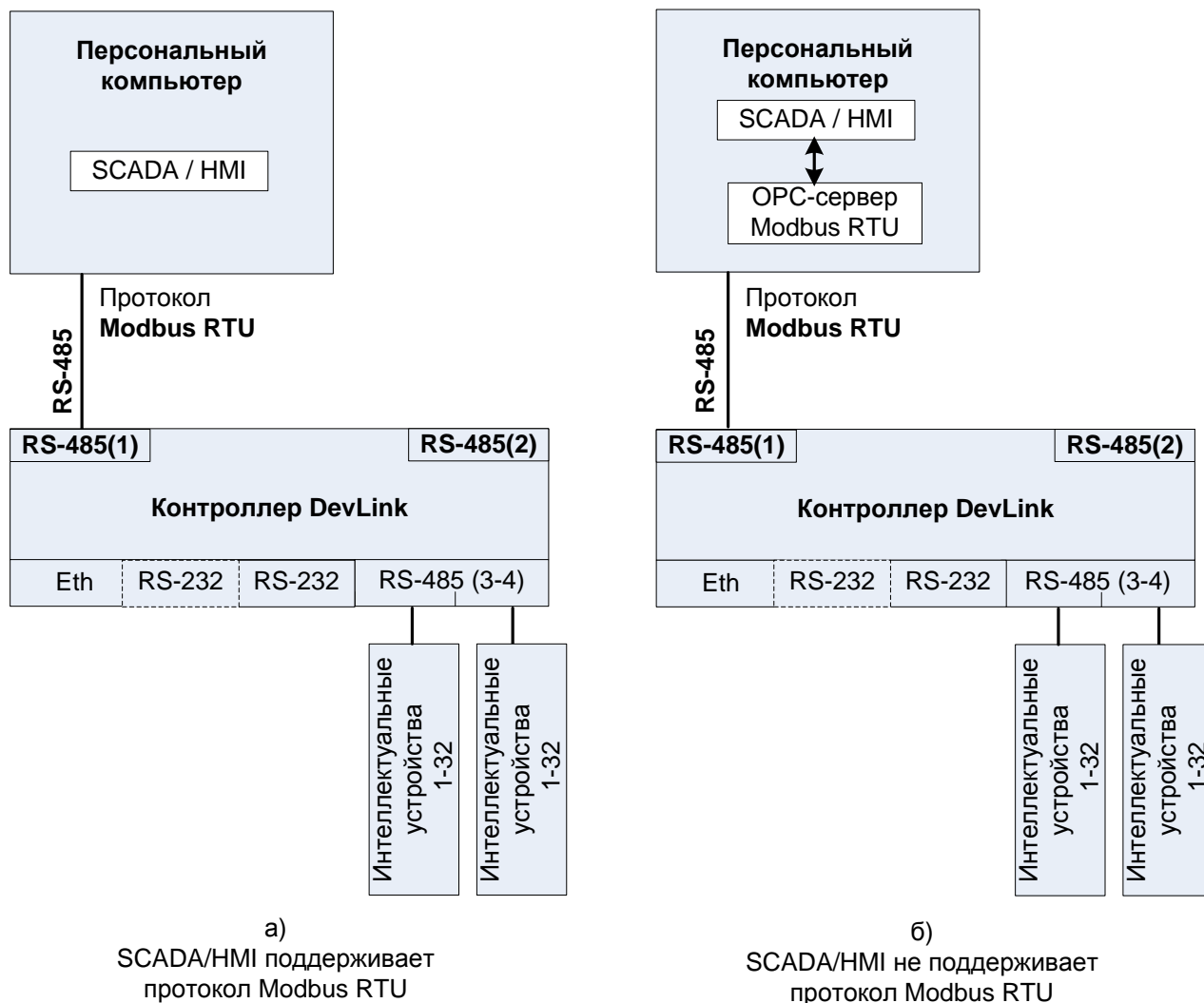
Рисунок 5.5 – Схема передачи данных по линии связи RS-485
