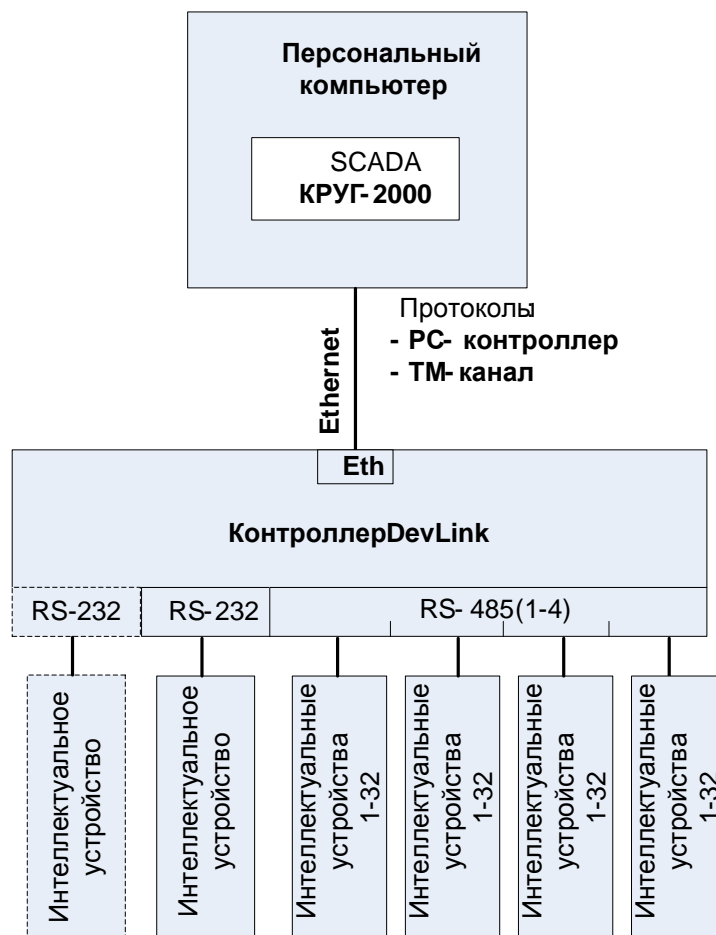
Рисунок 5.3 – Схема передачи данных по сети Ethernet по протоколу ТМ-канал
