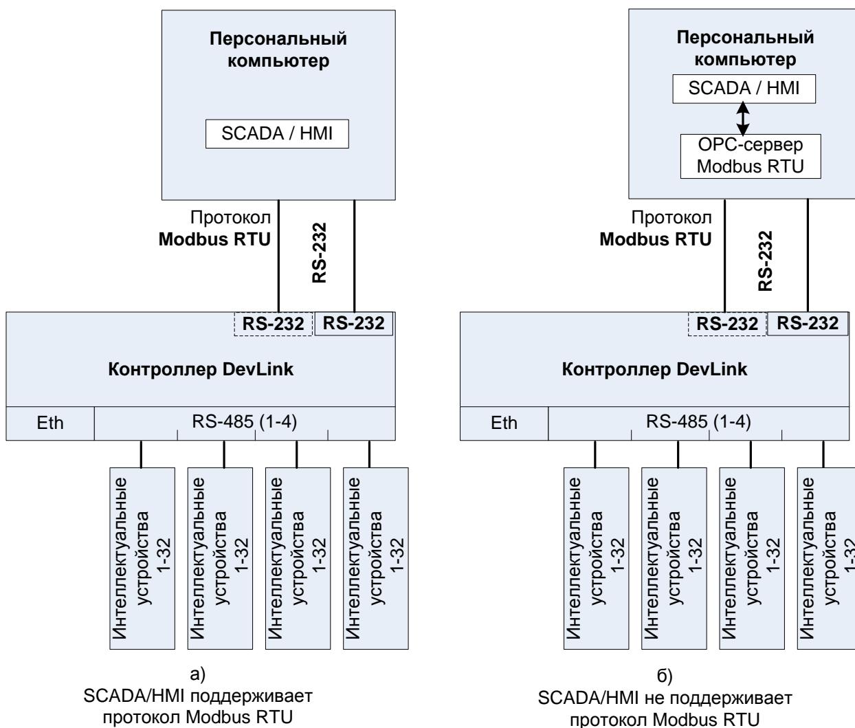
Рисунок 5.4 – Схема передачи данных по линии связи RS-232
