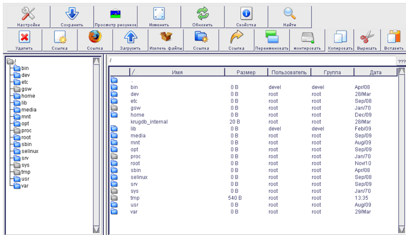
Рисунок 1.14 – Файловый менеджер
