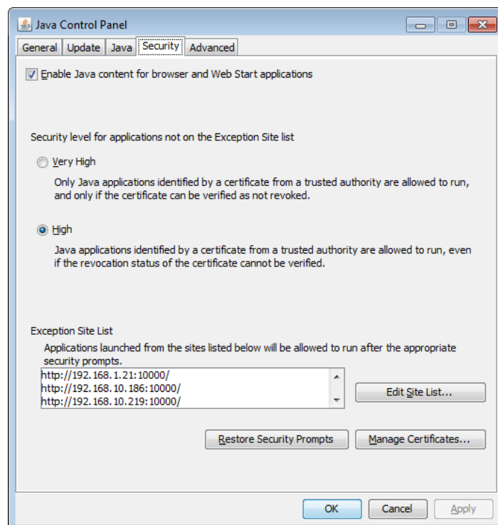
Рисунок 1.15 – Настройка Java-машины
