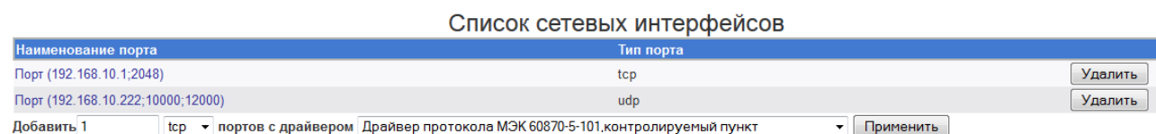
Рисунок 3.54 – Сетевые интерфейсы
