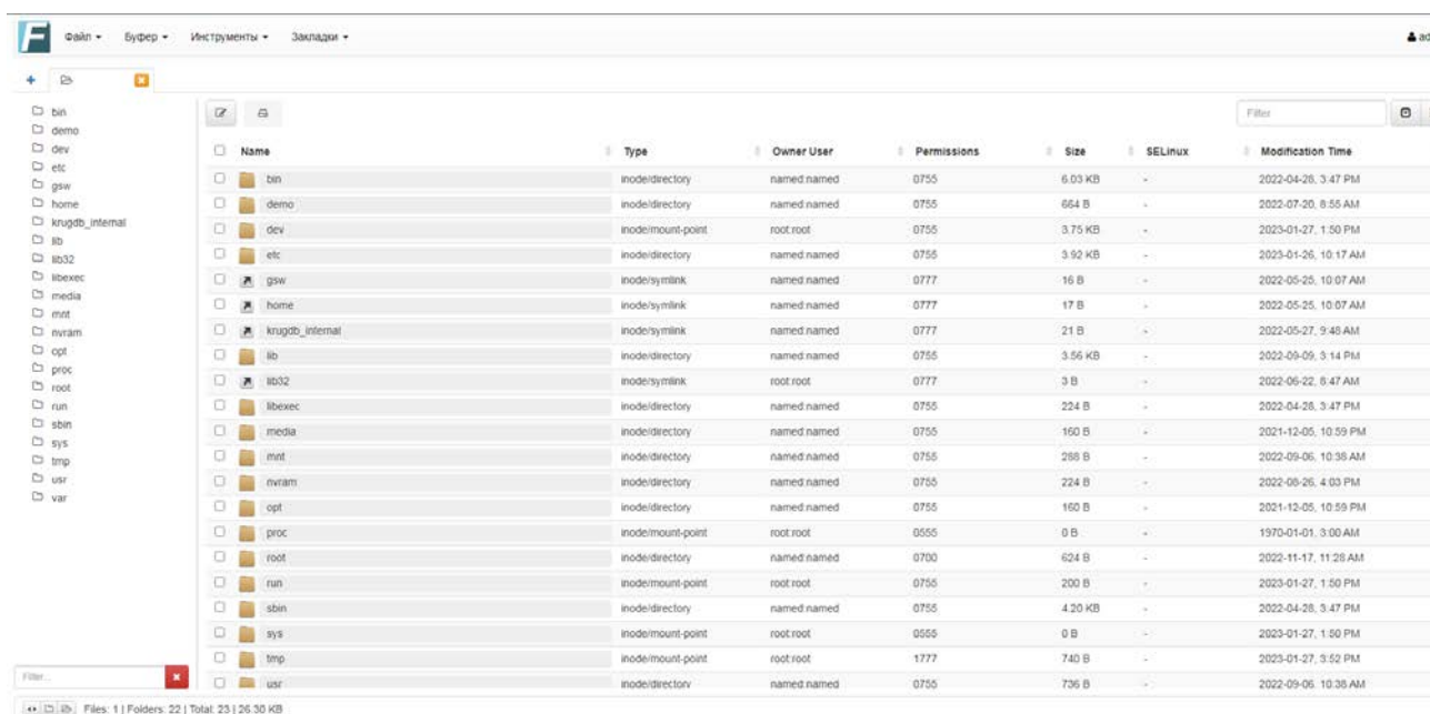
Рисунок 1.16 – Файловый менеджер
