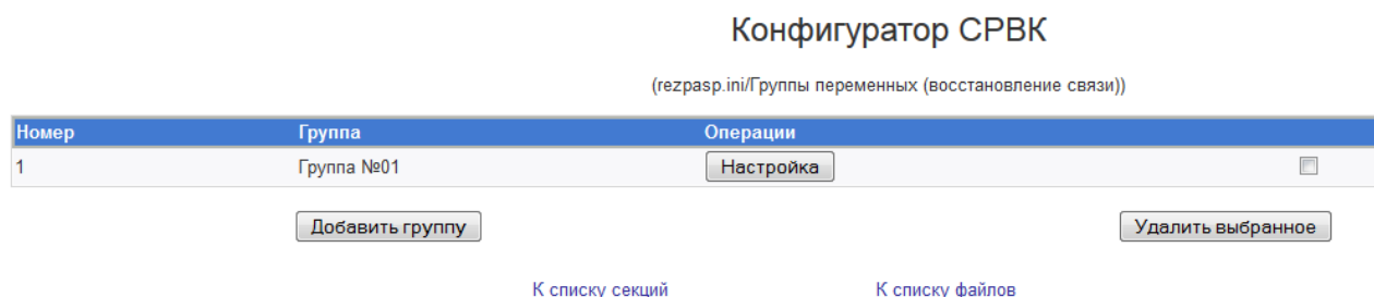
Рисунок 3.45 – Группы переменных
