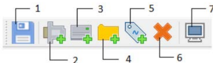
Рисунок 6.3 – Панель инструментов
