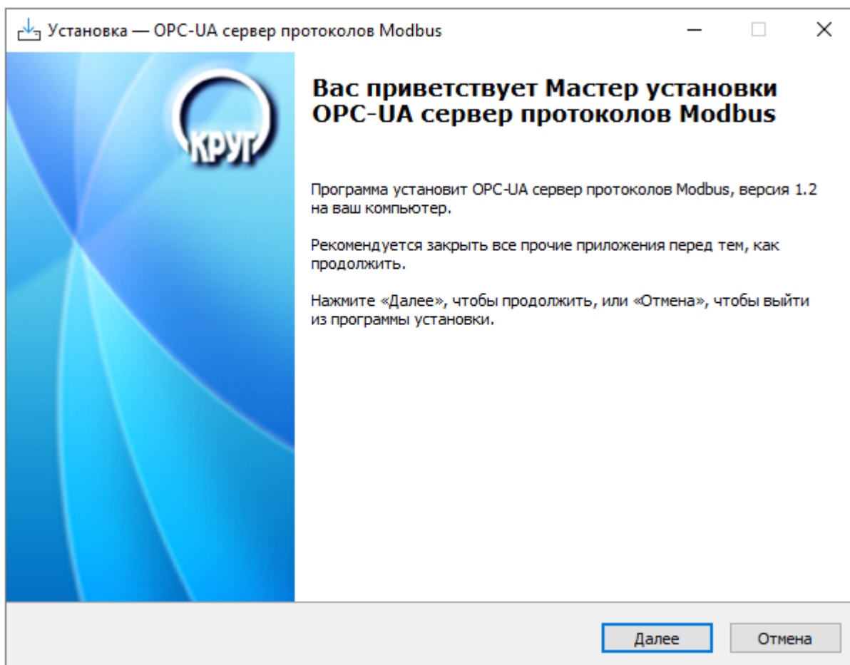
Рисунок 3.1 - Окно инсталлятора
