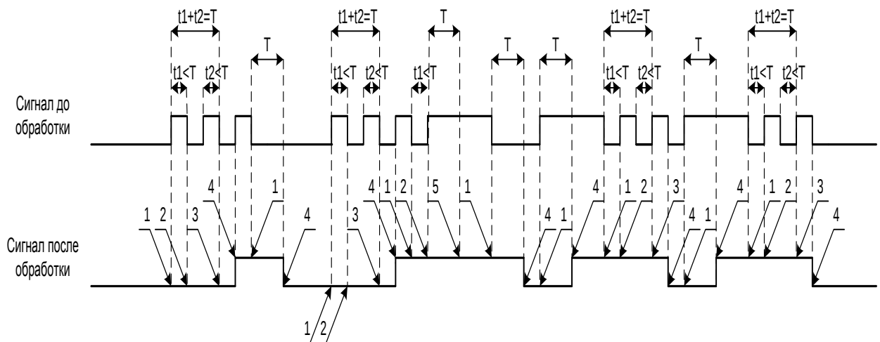
Рисунок J.2.4 - Фильтрация входного сигнала
