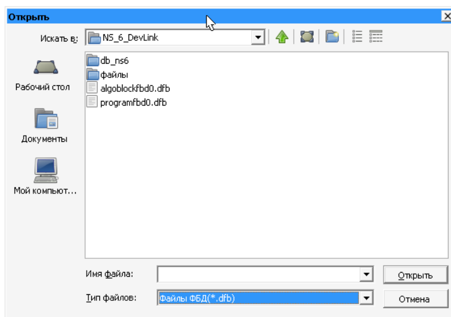
Рисунок 5.3.7 – Окно «Открыть»
