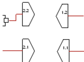
Рисунок 5.3.13 – Маркеры перехода
