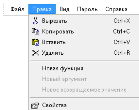
Рисунок 6.2.7 – Меню «Правка»
