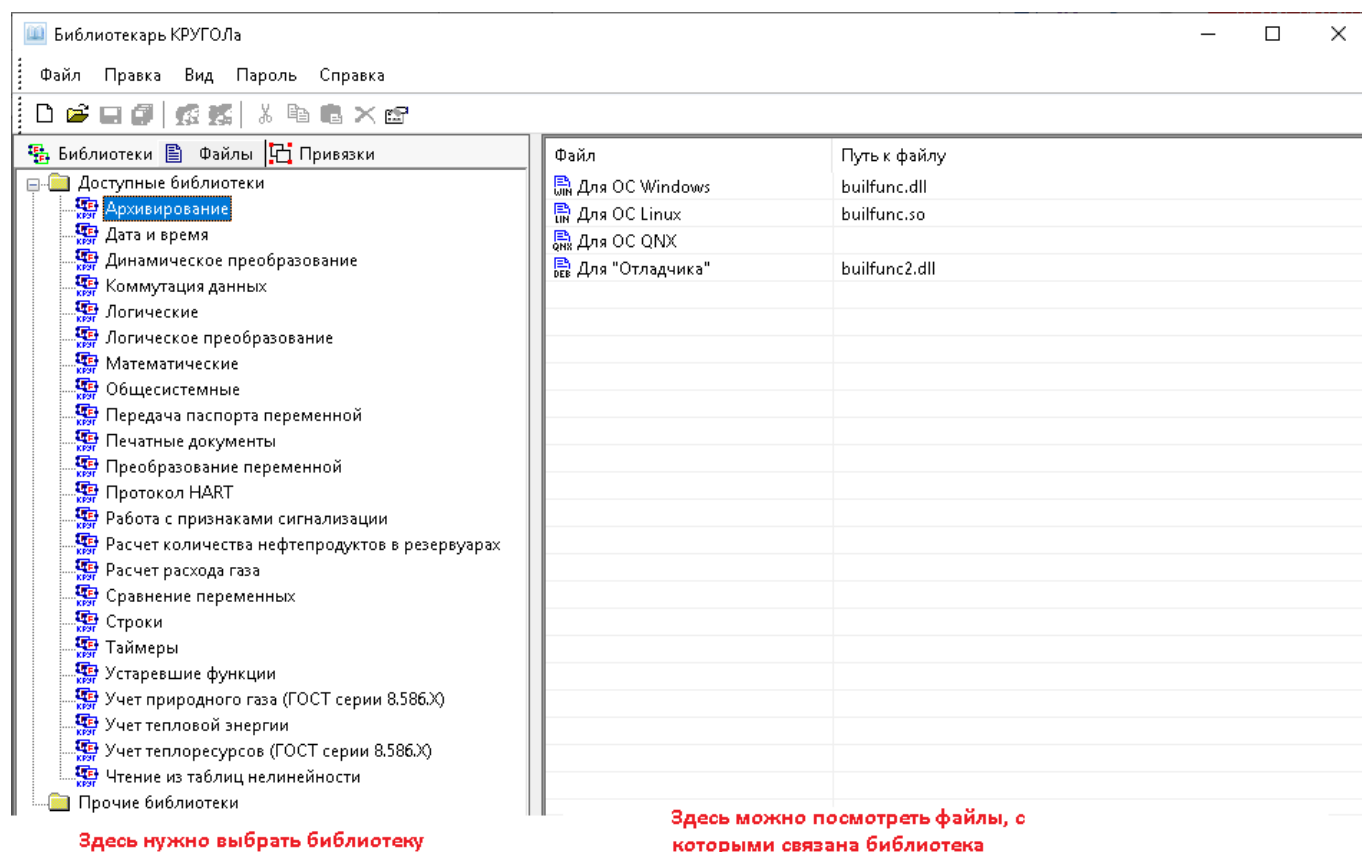
Рисунок 6.3.6 – Вкладка «Файлы»
