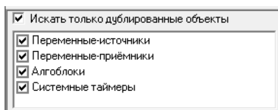
Рисунок 5.8.4 – «Дублированные объекты»
