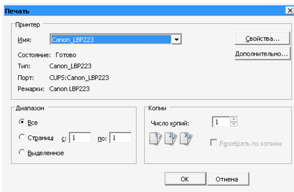
Рисунок 5.3.10 – Окно «Печать»
