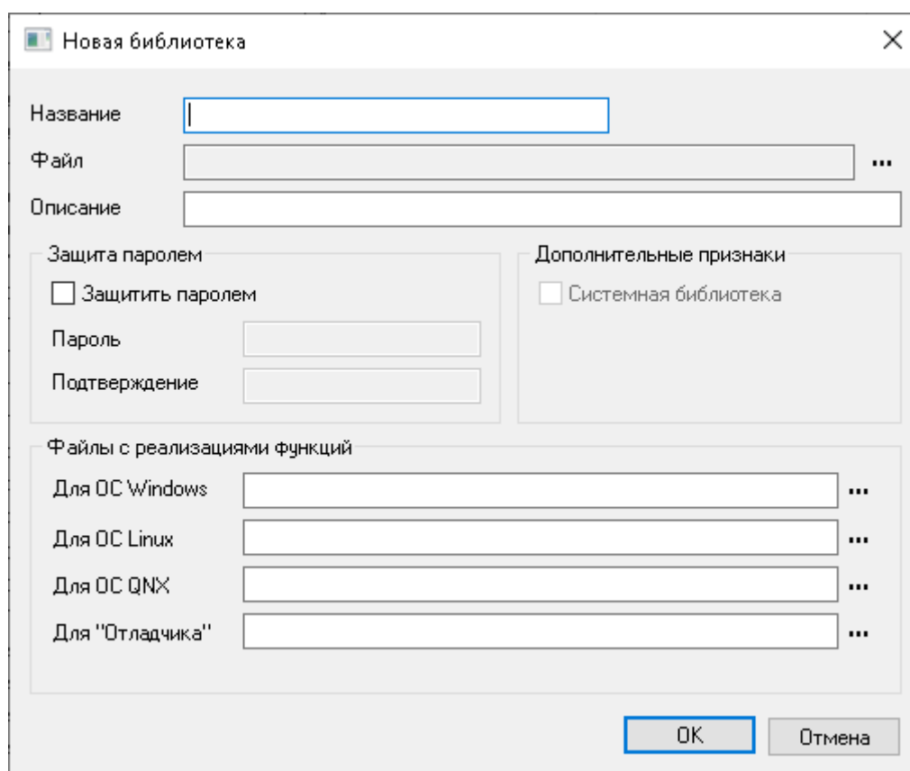
Рисунок 6.2.4 – Параметры библиотеки
