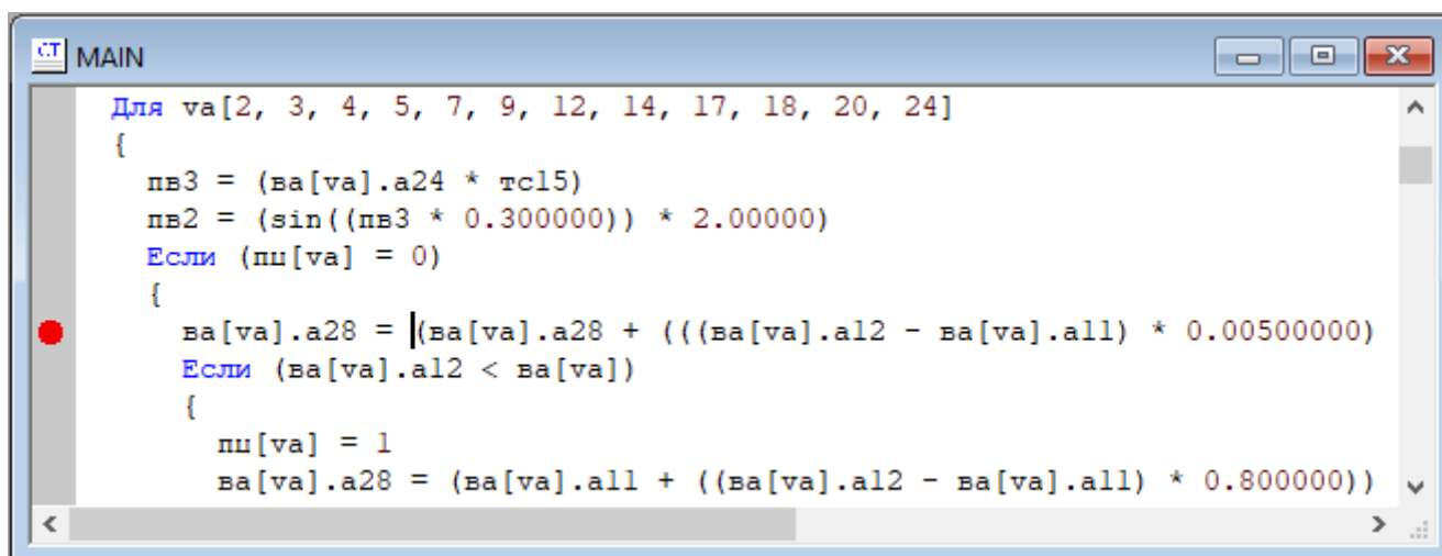
Рисунок 5.4.4 – Точка останова
