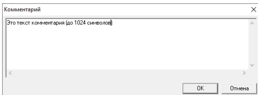
Рисунок 5.4.11 – Окно «Комментарий»
