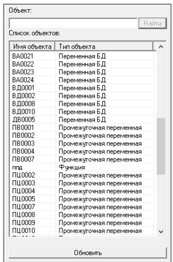
Рисунок 5.8.5 – «Найденные объекты»
