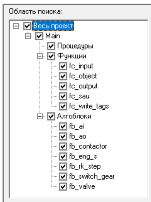
Рисунок 5.8.2 – «Область поиска»
