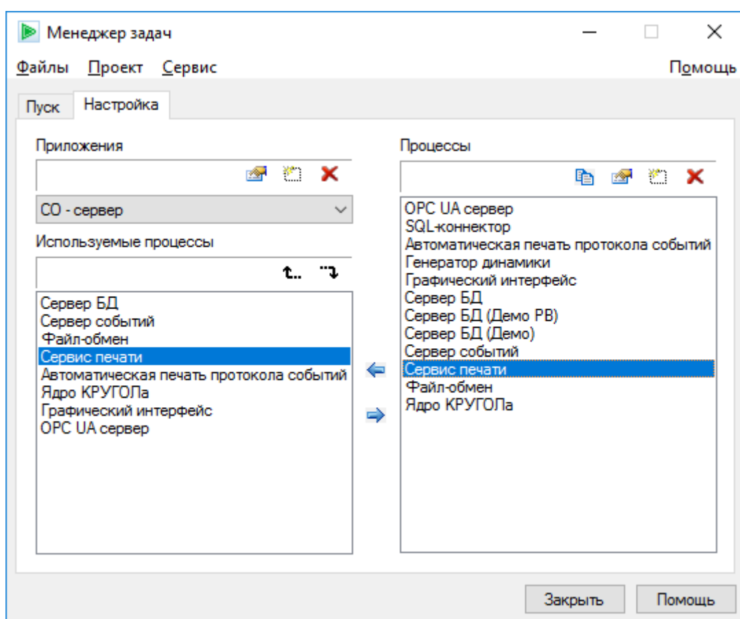
Рисунок 1.3.1 - Добавление процесса «Сервис печати» в приложение
