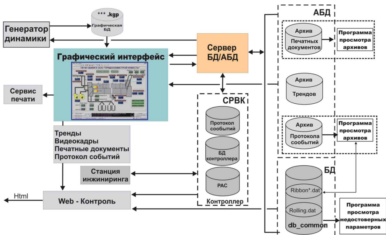
Рисунок 1.2.1 – Графический интерфейс в Среде исполнения
