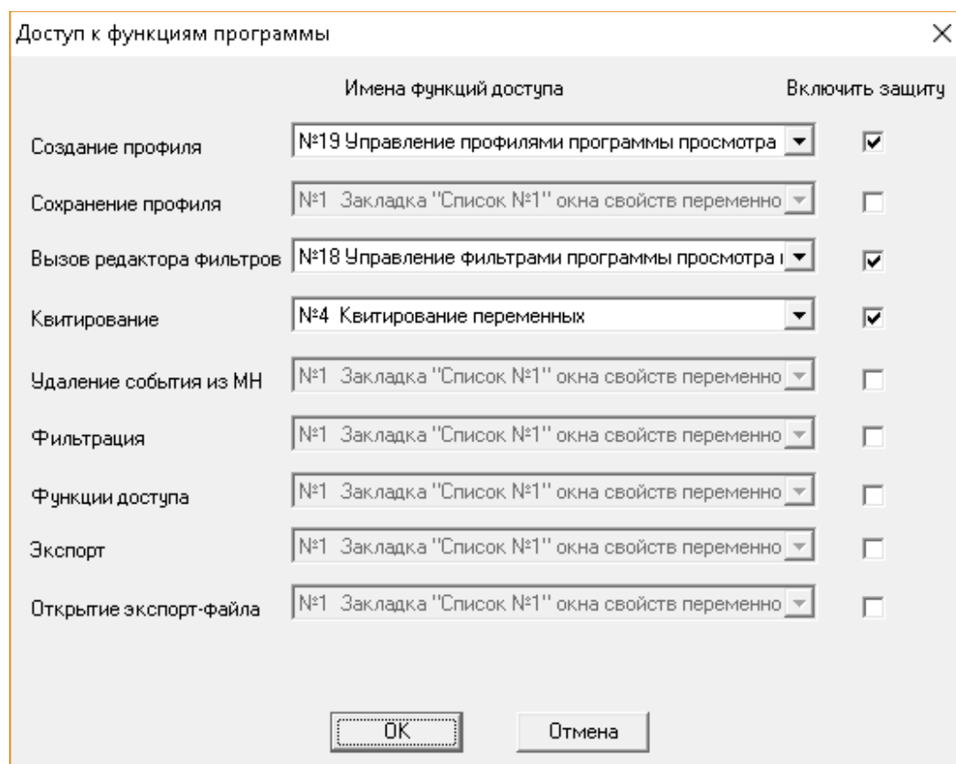
Рисунок 1.6.15 - Диалог настроек доступа к функциям программы
