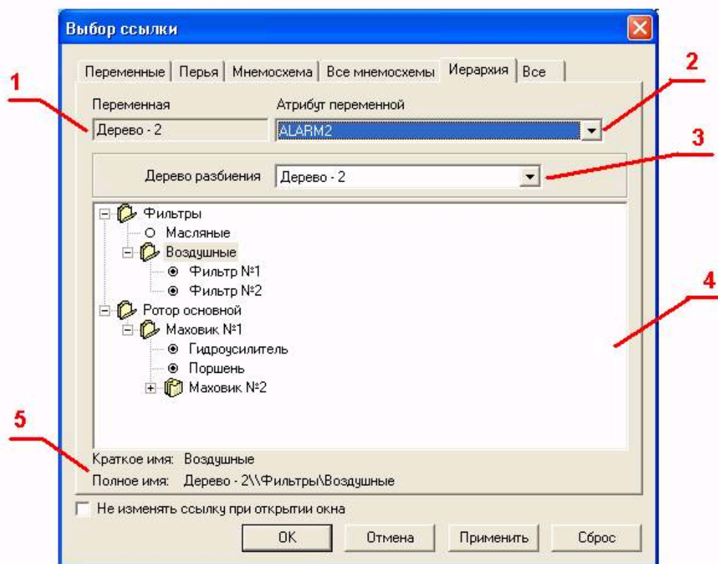
Рисунок 1.8.9 - Окно выбора ссылок. Закладка «Иерархия»
