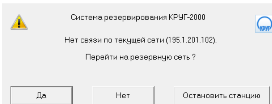
Рисунок 3.5.4 - Окно предупреждения при отсутствии связи с сервером по текущей сети
