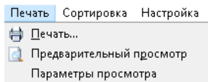
Рисунок 1.6.6 - Подменю «Печать»
