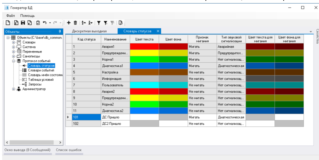
Рисунок 1.6.11 - Настройка цвета мигания текстом/фоном
