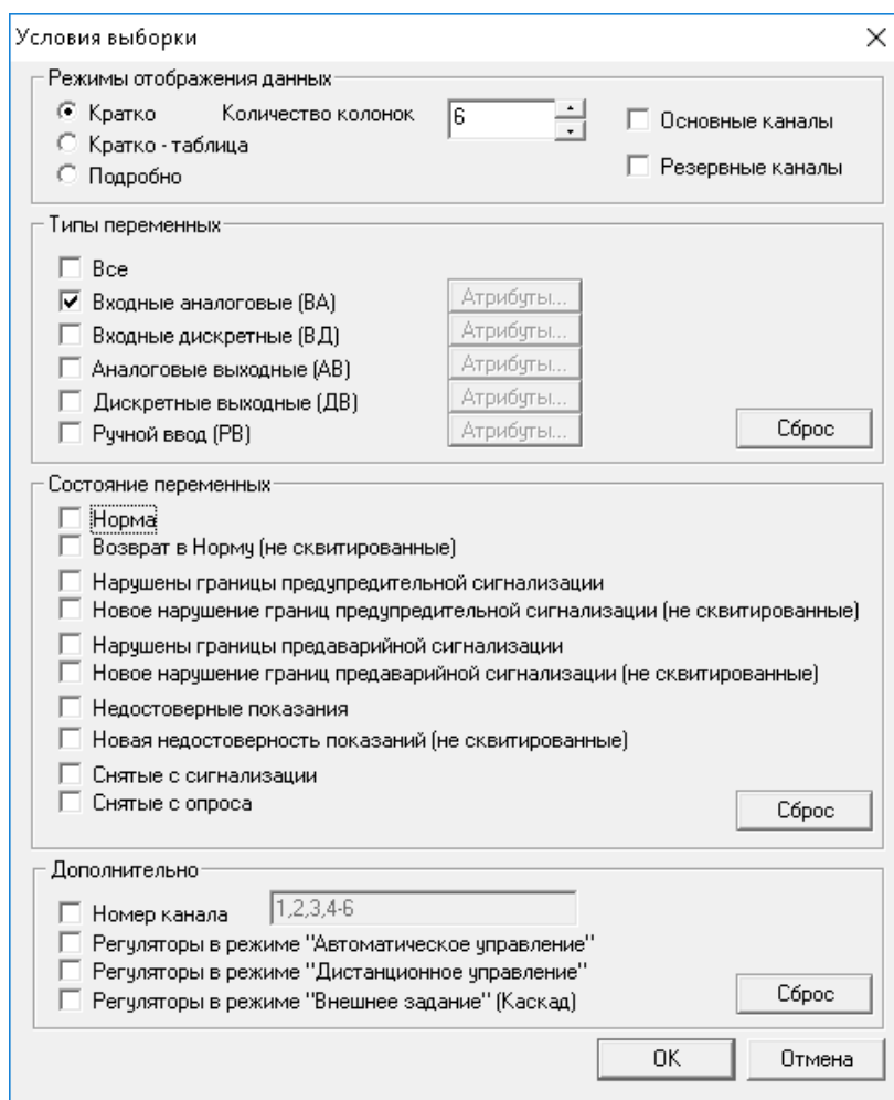
Рисунок 1.9.6 - Окно «Условия выборки»
