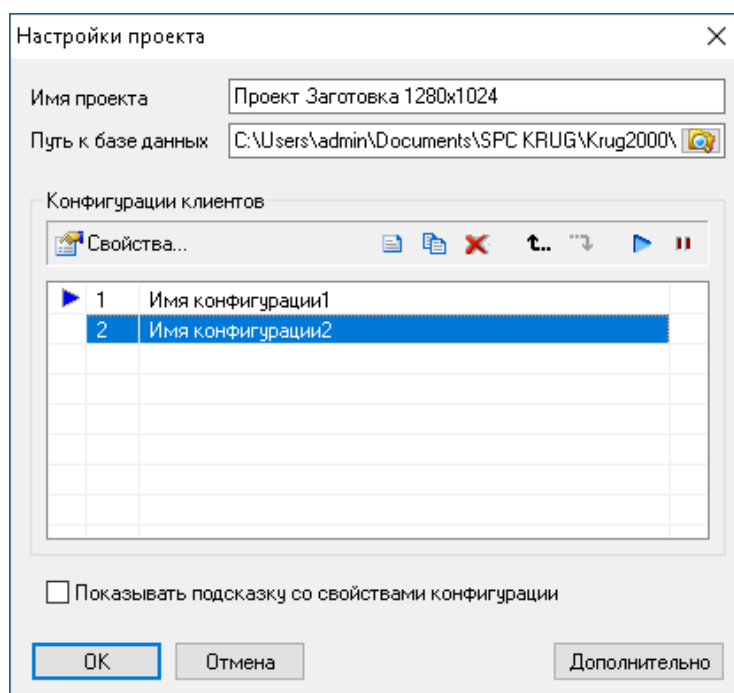
Рисунок 3.3.2 - Элементы настройки конфигурации клиента
