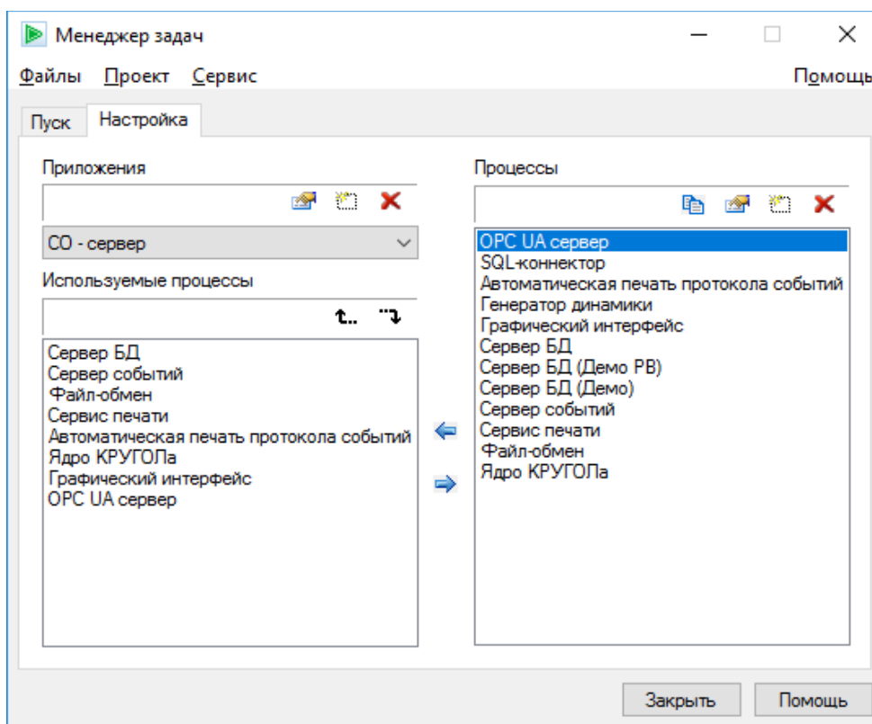
Рисунок 3.2.1 - Настройка параметров запуска приложений
