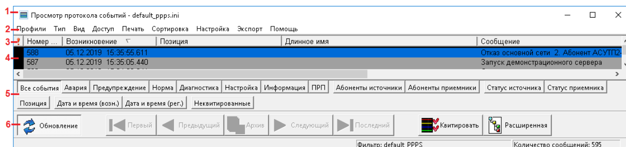
Рисунок 1.6.1 - Главное окно программы «Просмотр протокола событий»
