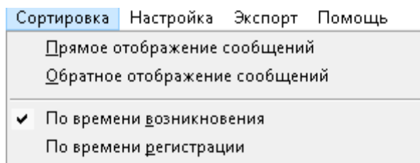
Рисунок 1.6.9 - Подменю «Сортировка»
