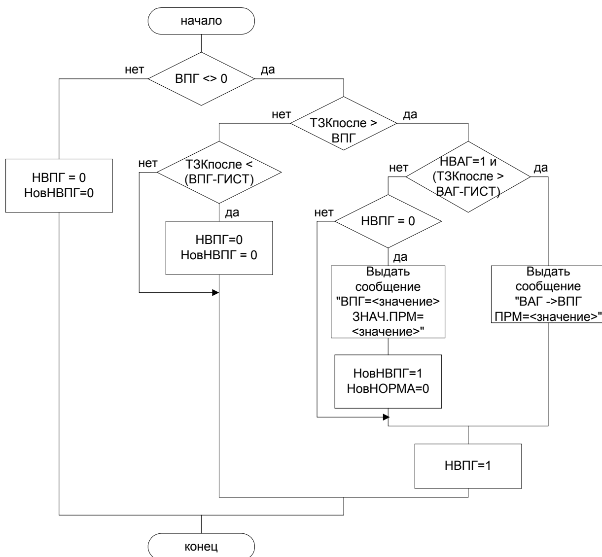
Рисунок 3.10.4 - Алгоритм обработки Верхней Предупредительной Границы
