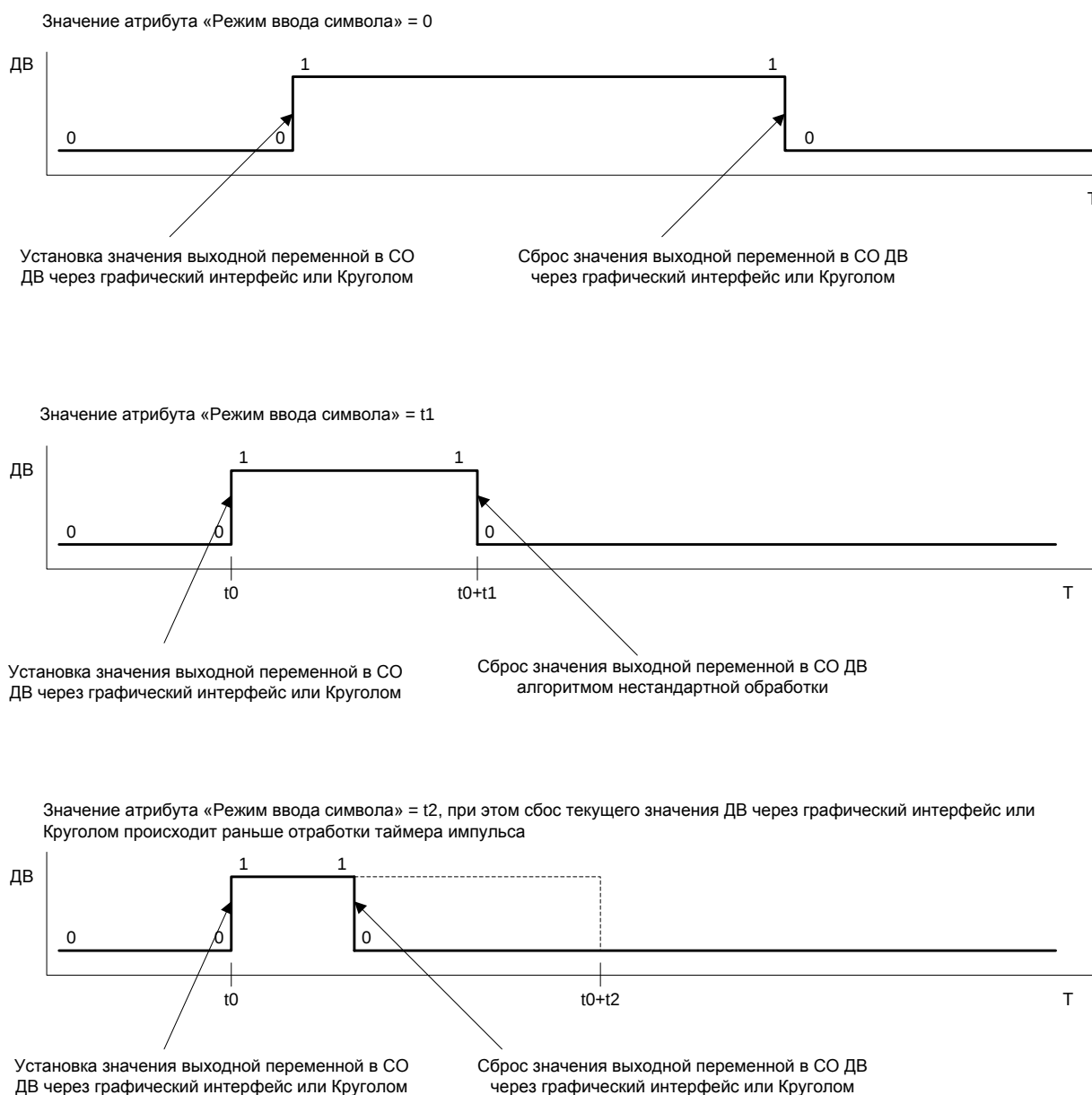
Рисунок 3.10.12 - Пример использования режима ввода символа по алгоритму №3
