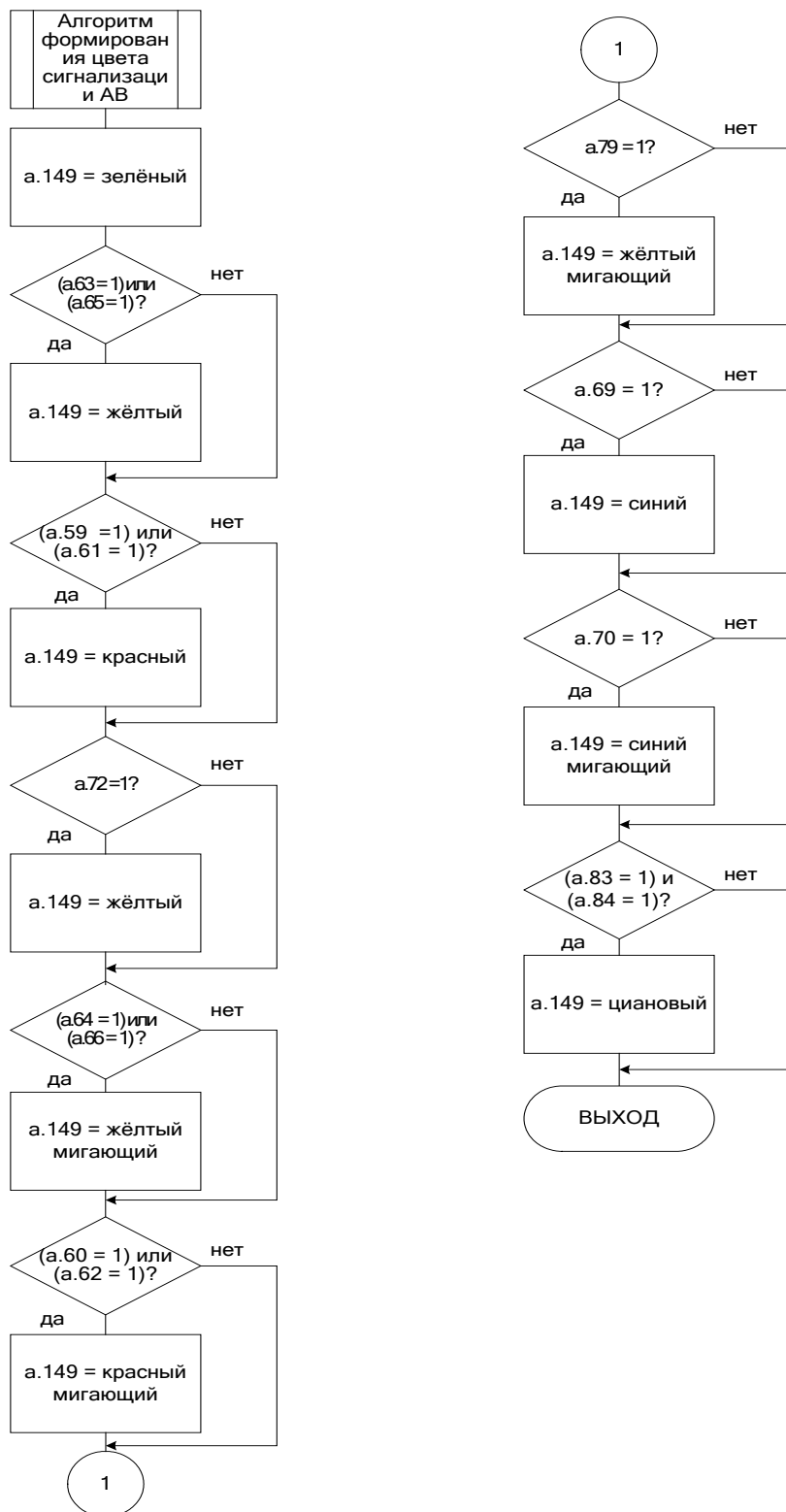
Рисунок 3.10.8 - Блок-схема алгоритма формирования цвета сигнализации
