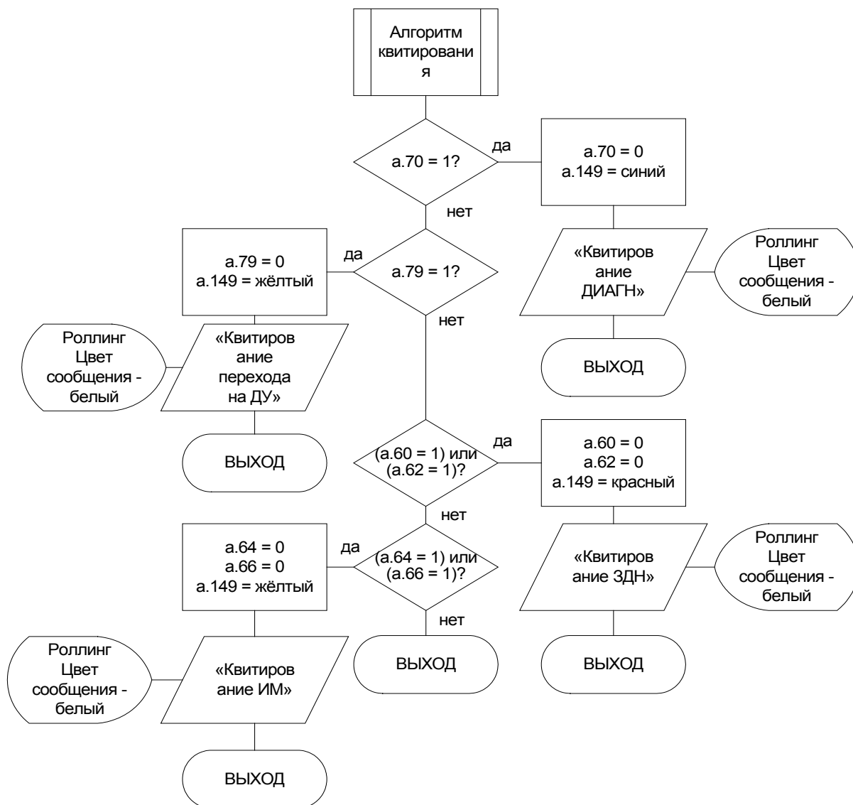
Рисунок 3.10.9 - Блок-схема алгоритма квитирования сигнализации
