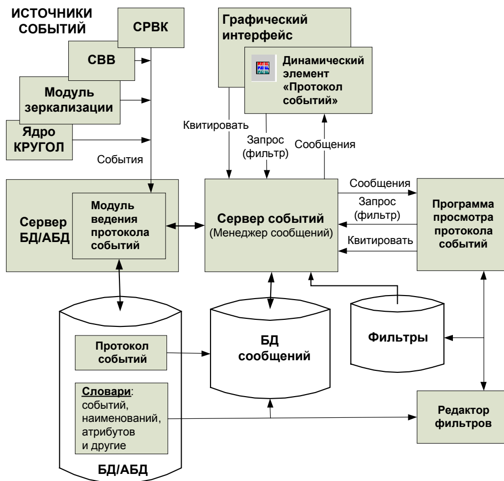
Рисунок 8.2.1 – Обработка и визуализация событий
