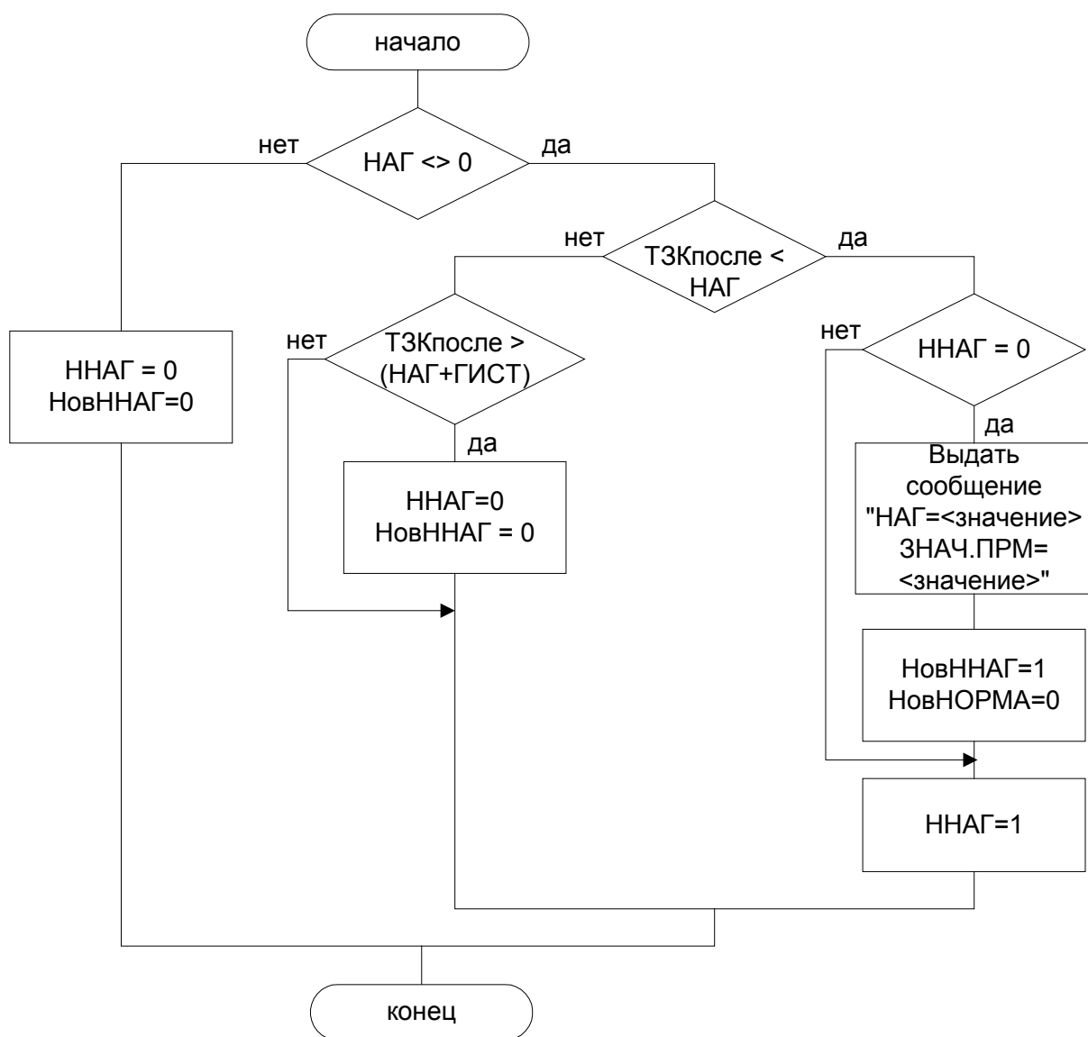
Рисунок 3.10.5 - Алгоритм обработки Нижней Предаварийной Границы
