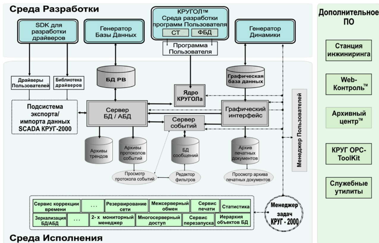
Рисунок 1.1.1 - Архитектура среды исполнения
