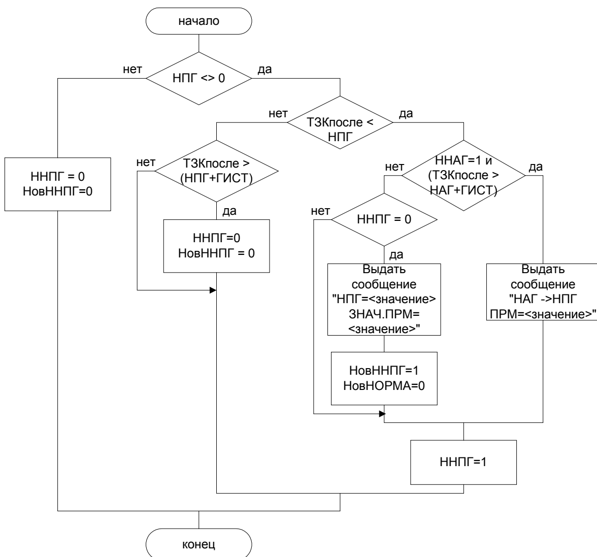
Рисунок 3.10.3 - Алгоритм обработки Нижней Предупредительной Границы
