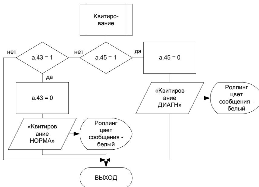
Рисунок 3.10.15 - Блок-схема квитирования для алгоритмов №1, №2 и №3 нестандартной обработки ДВ переменной
