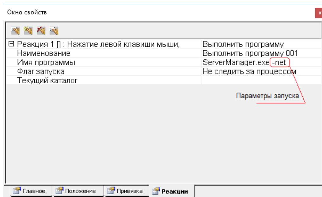
Рисунок 11.1 – Окно свойств
