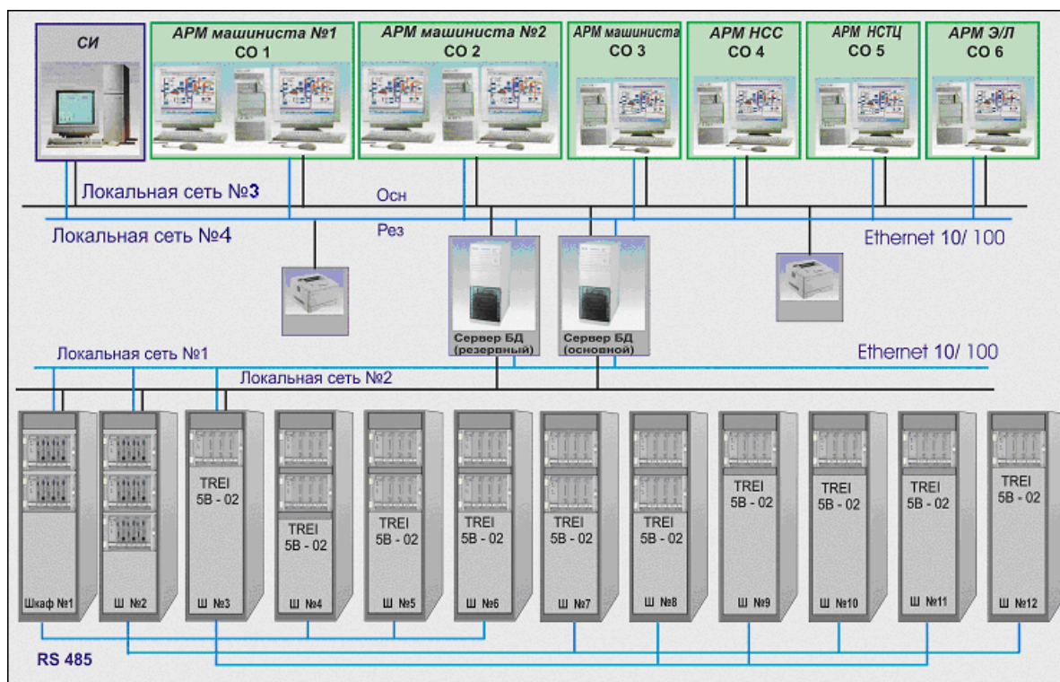
Рисунок 2.5.1 - PCY на базе КРУГ-2000
