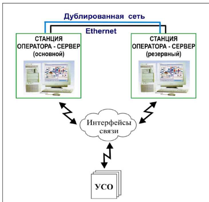
Рисунок 2.3.1 - Схема с резервированием серверов
