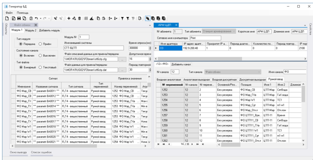
Рисунок 3.10 – Настройка модуля Файл-обмен и описание канала «Файл-Обмен», в котором осуществляется формирование атрибутов переменных
