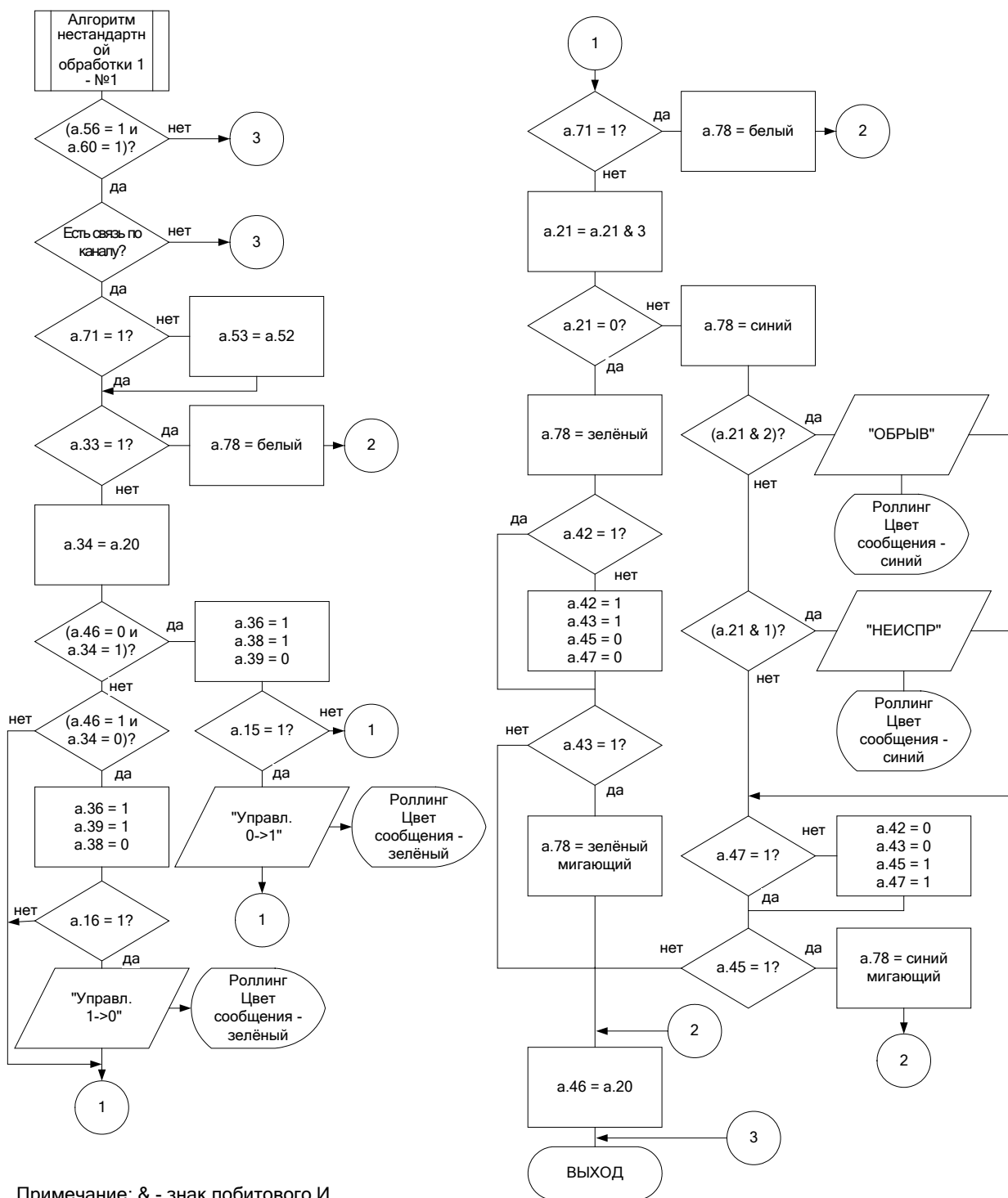
Рисунок 3.10.13 - Блок-схема алгоритма №1 нестандартной обработки ДВ
