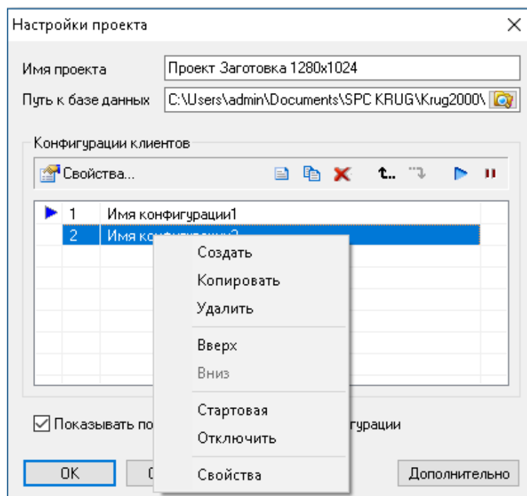
Рисунок 10.3 - Окно «Настройки проекта» с операциями над конфигурациями
