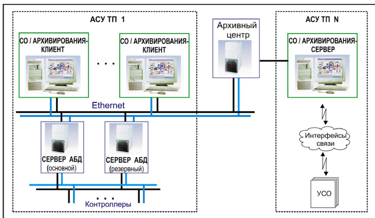
Рисунок 2.7.2 - Архивный центр в архитектуре АСУ ТП верхнего уровня
