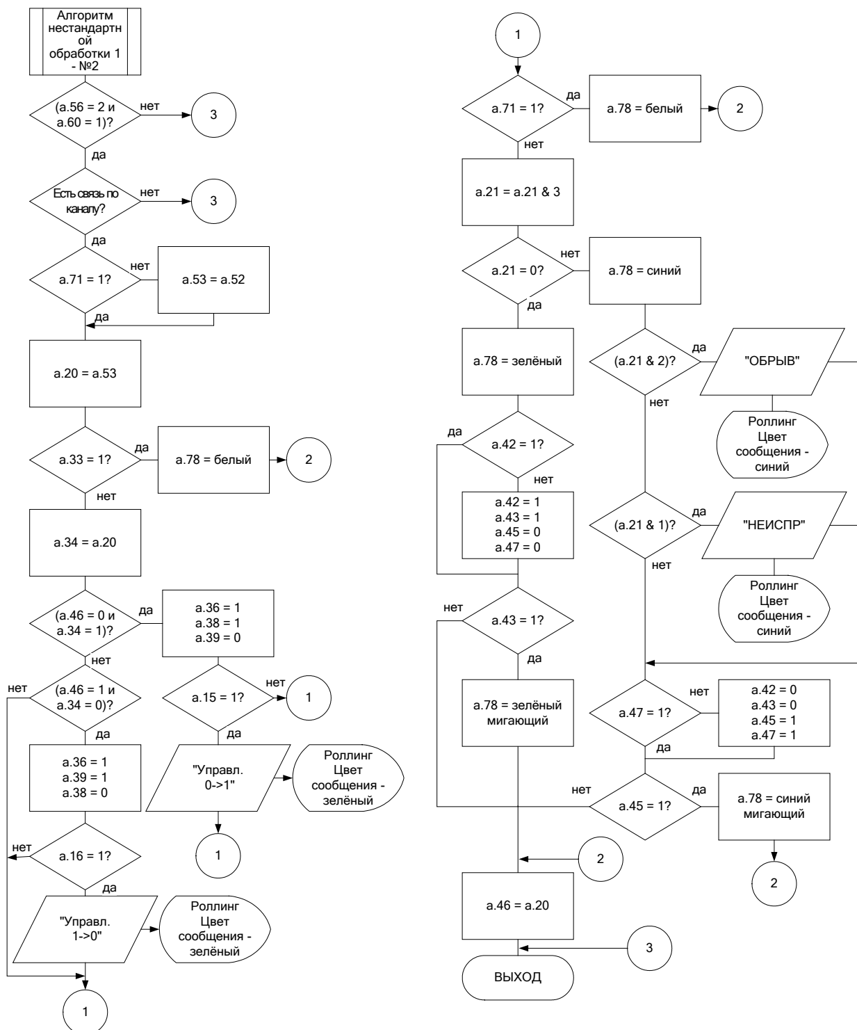
Рисунок 3.10.14 - Блок-схема алгоритма №2 нестандартной обработки ДВ
