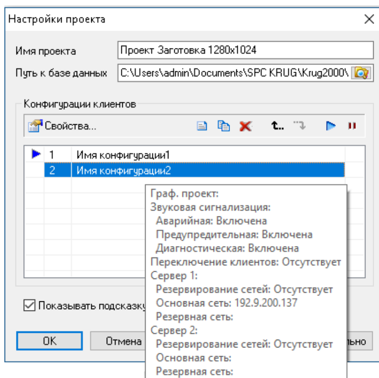
Рисунок 10.2 - Окно «Настройки проекта» с кратким описанием параметров конфигурации
