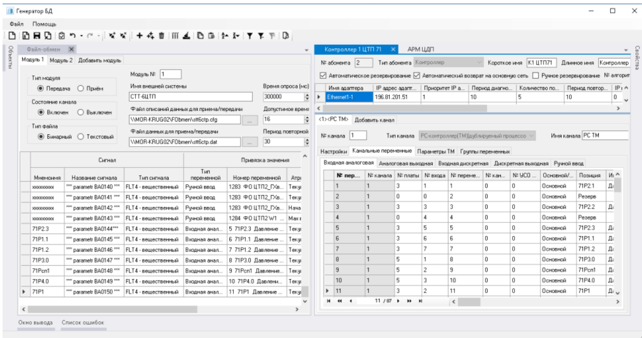
Рисунок 3.11 – Настройка модуля Файл-обмен и описание канала «PC-контроллер (TM) (дублируемый процессор)», в котором осуществляется формирование атрибутов переменных
