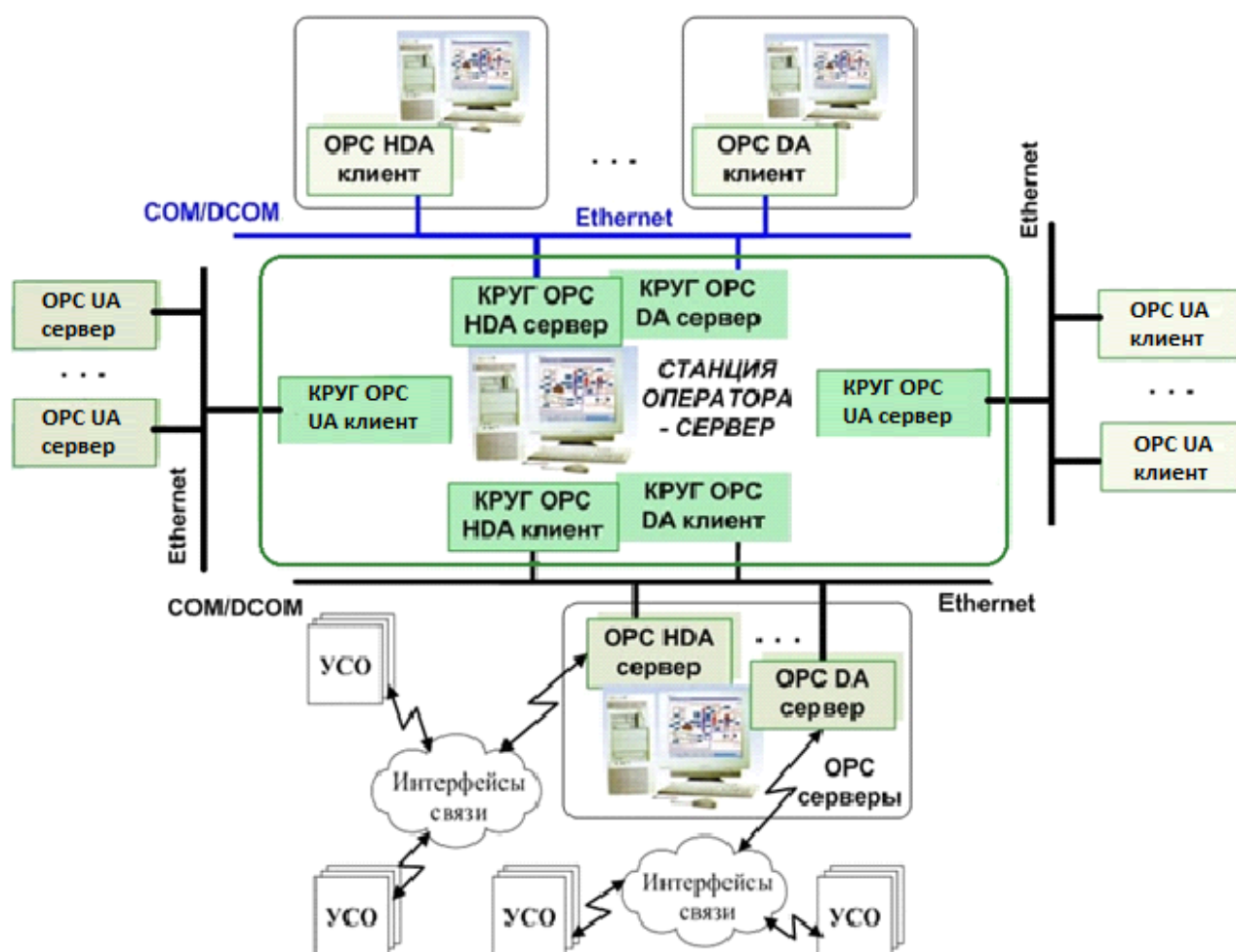
Рисунок 2.6.1 – Структура системы управления на основе OPC-технологии
