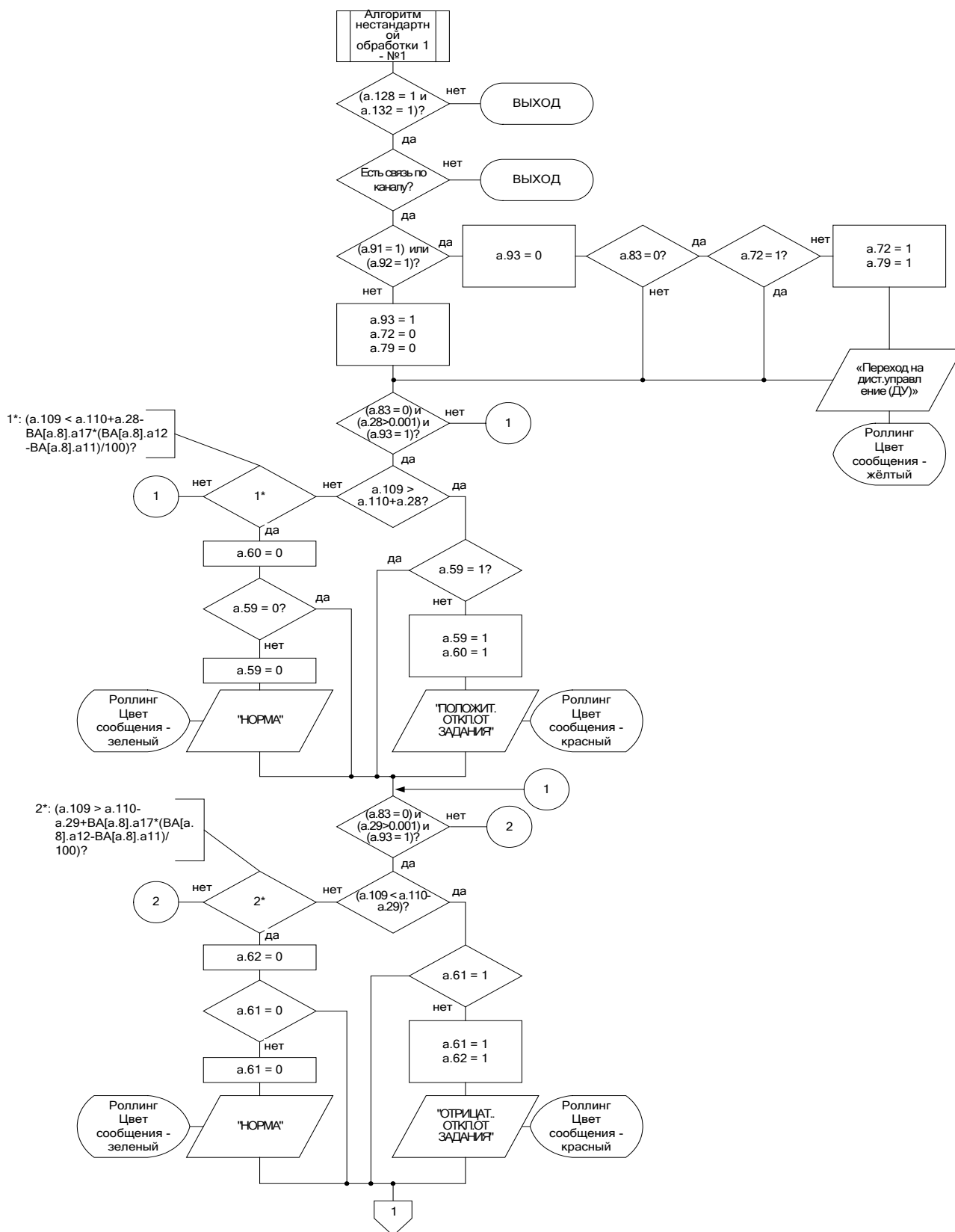
Рисунок 3.10.7 - Блок-схема алгоритма №1 нестандартной обработки АВ переменной
