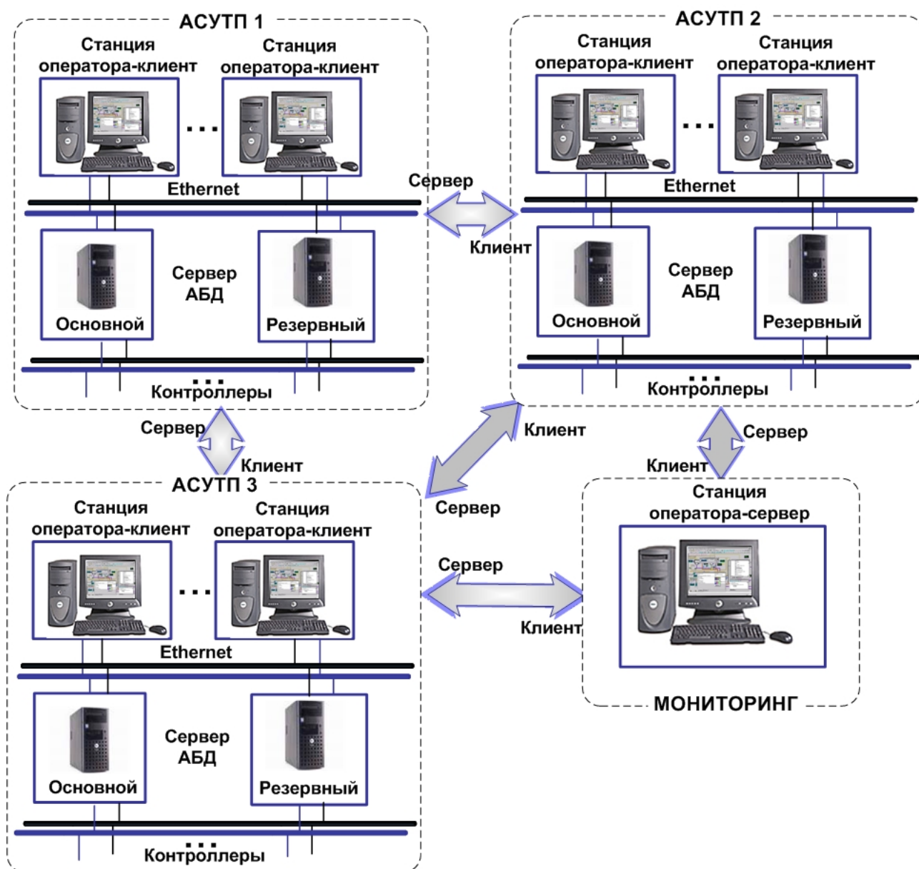
Рисунок 9.1.1 – Архитектура межсерверного обмена
