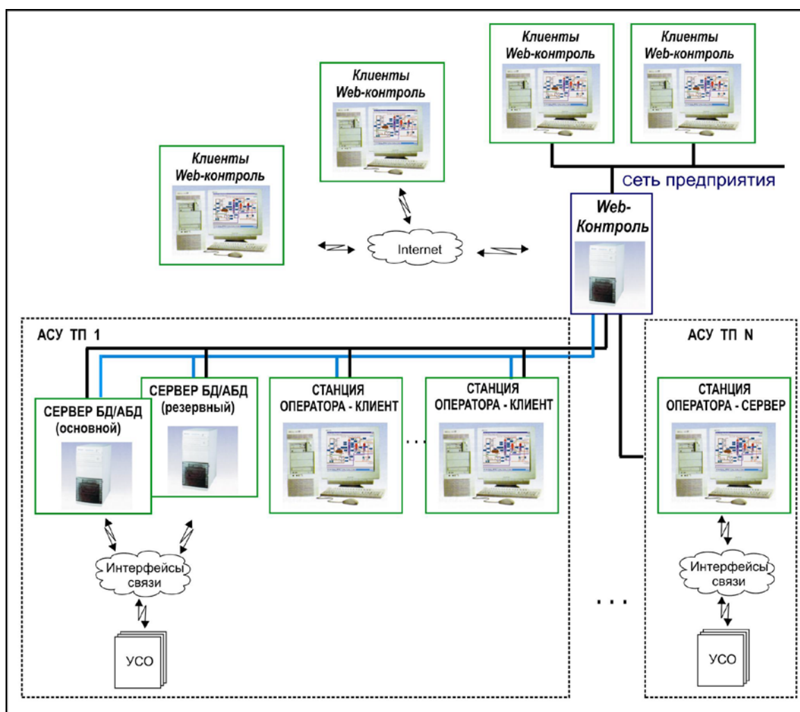
Рисунок 2.7.1 - Web-Контроль в архитектуре верхнего уровня АСУ ТП
