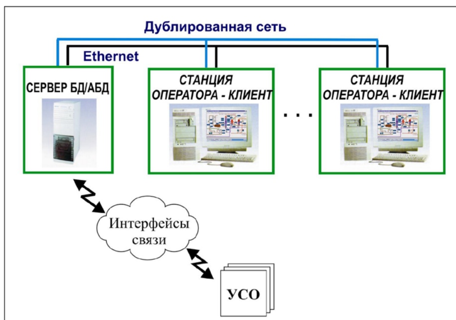
Рисунок 2.2.1 - Схема клиент-сервер
