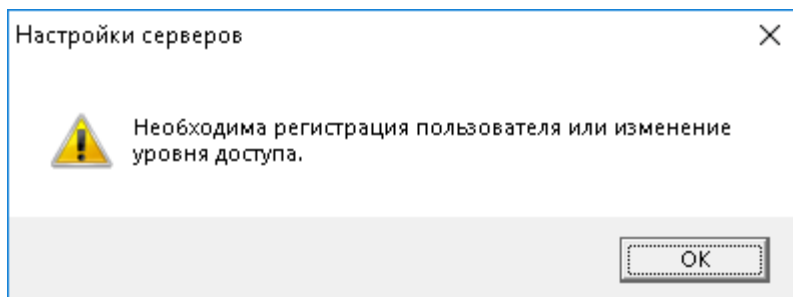
Рисунок 11.4 Окно сообщения
