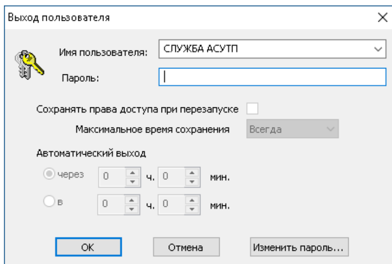
Рисунок 11.11 - Выход Пользователя
