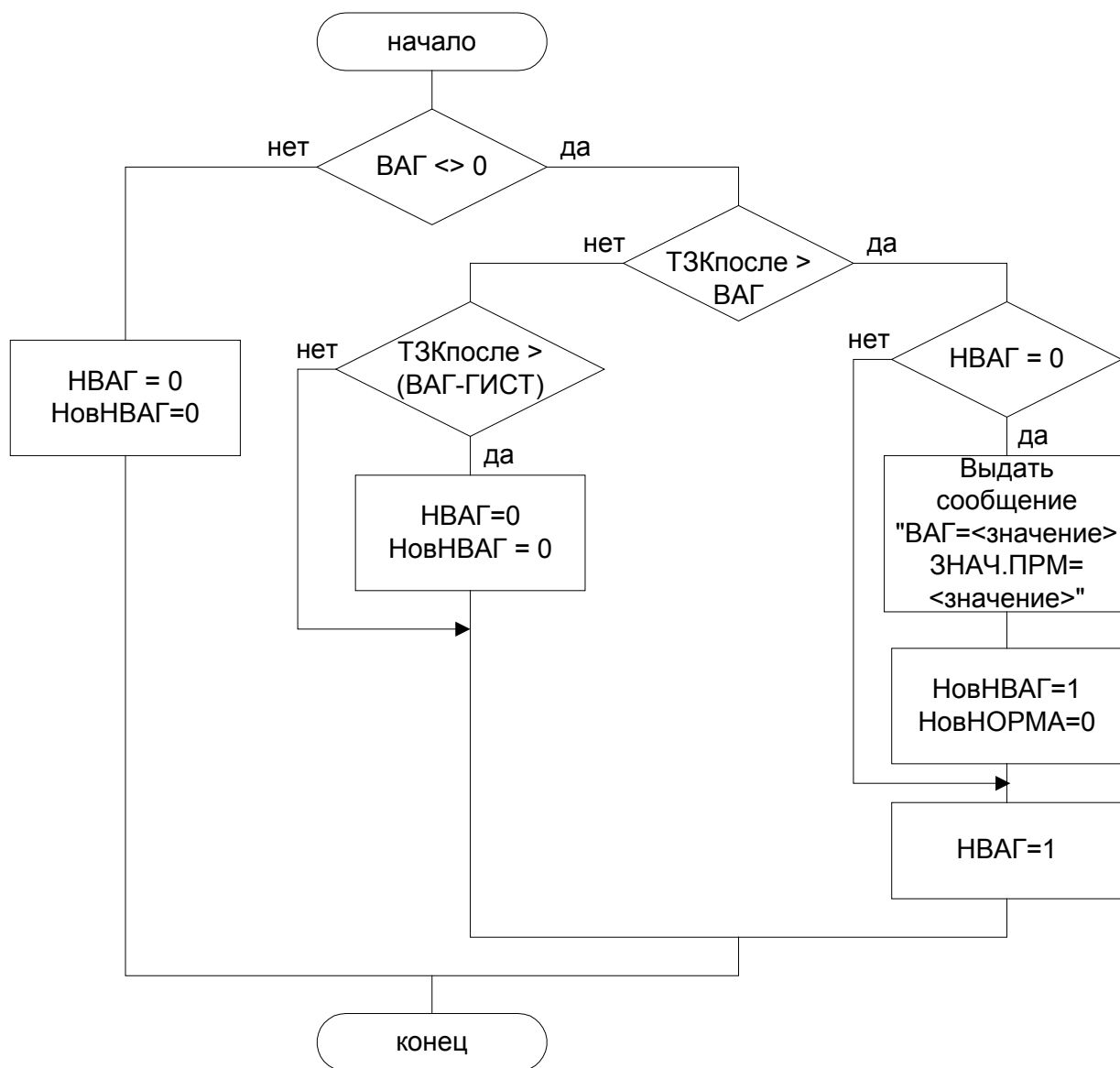
Рисунок 3.10.6 - Алгоритм обработки Верхней Предаварийной Границы
