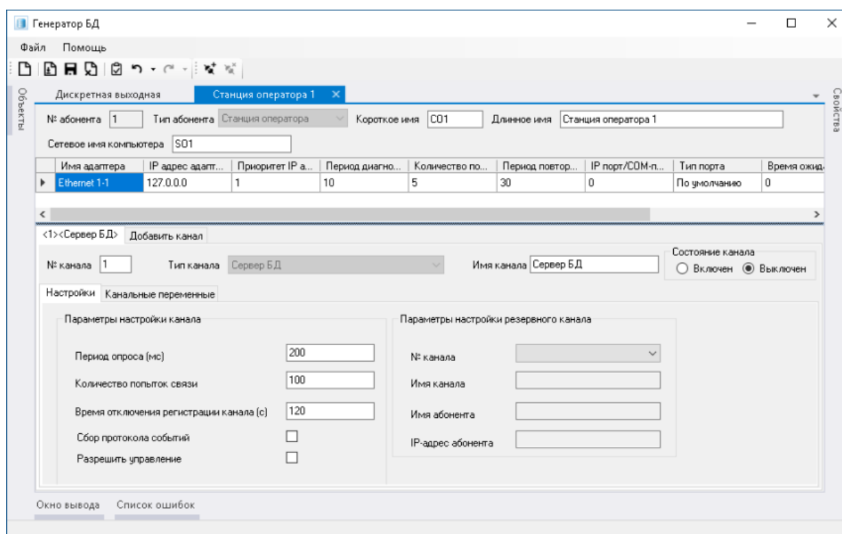
Рисунок 9.3.1 – Настройка канала «Сервер БД» в Генераторе базы данных
