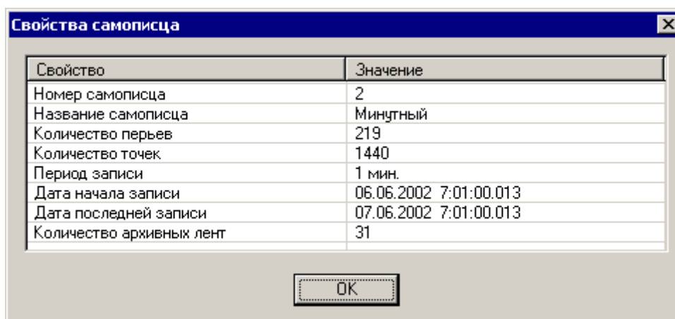
Рисунок 5.7 – Свойства самописца
