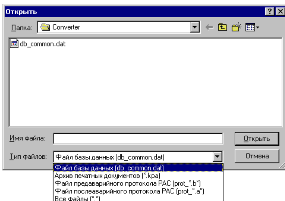
Рисунок 3.1 - Окно «Открыть»
