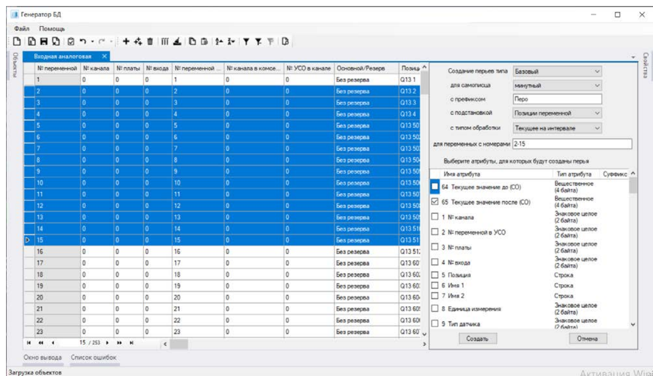
Рисунок 5.8.1 – Создание перьев самописцев с помощью трендрования переменных
