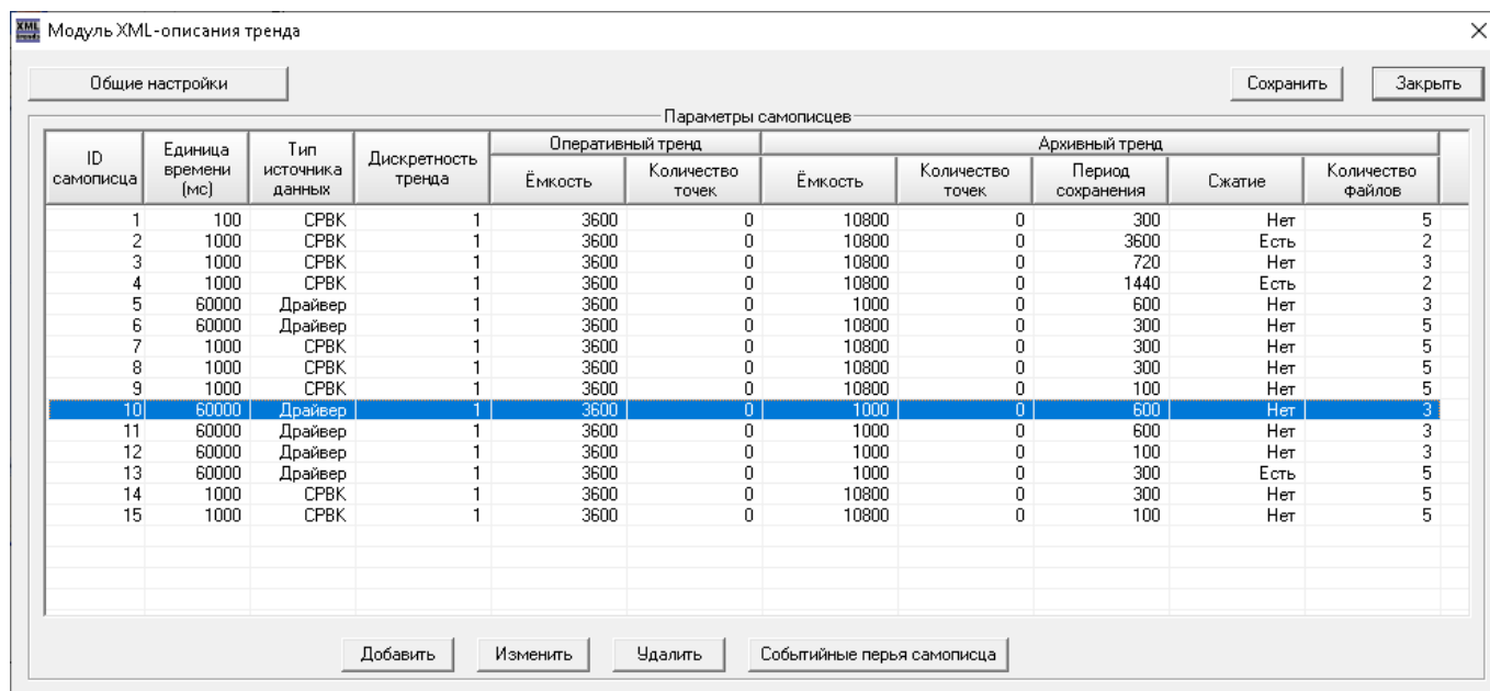
Рисунок 5.10.1– Главное окно Модуля XML-описания тренда
