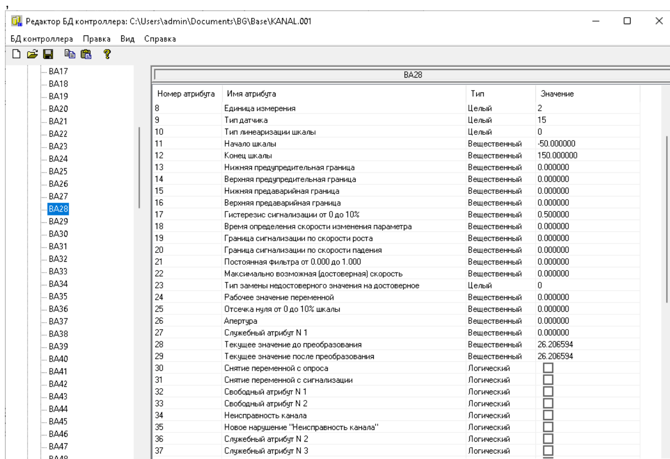
Рисунок 5.9.5 – Изменение паспорта переменной
