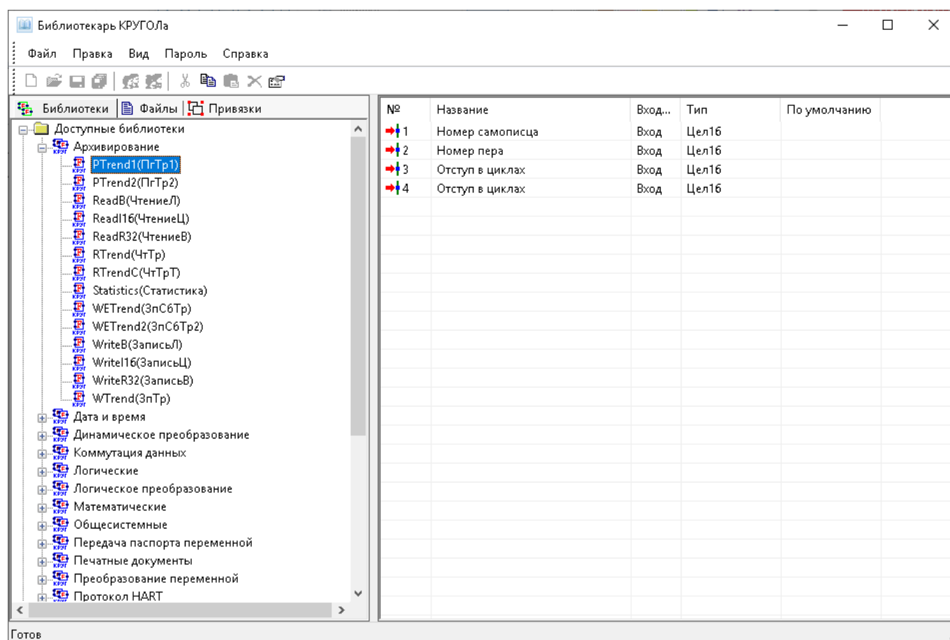
Рисунок 6.3.5 – Информация об аргументах функции
