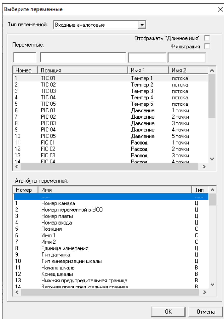
Рисунок 5.4.9 – Окно «Выберите переменные»
