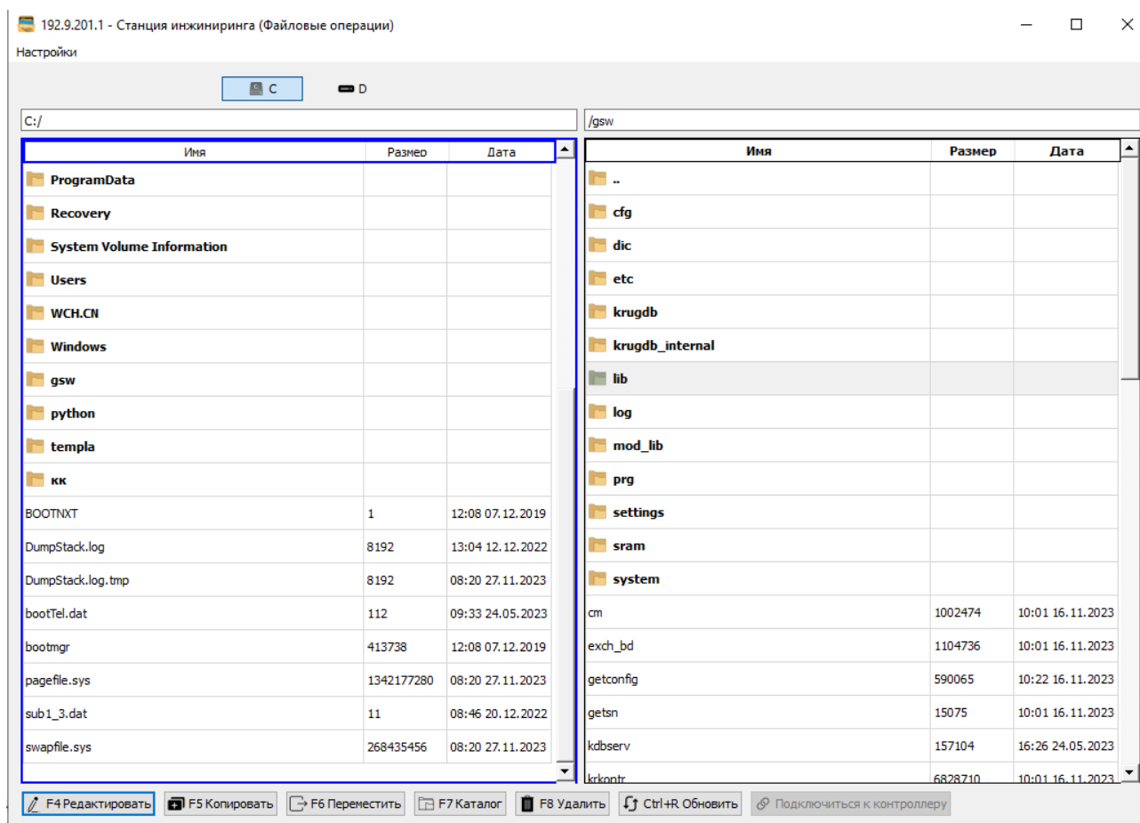
Рисунок 3.2 - Видеокادر работы с оболочкой файловых операций (для абонентов типа «Контроллер (тип 2)»)
